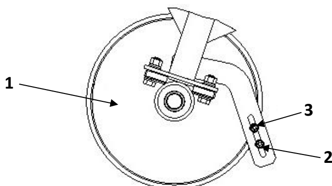
Rys. 7. Regulacja ustawienia skrobaka wału ugniatającego.
