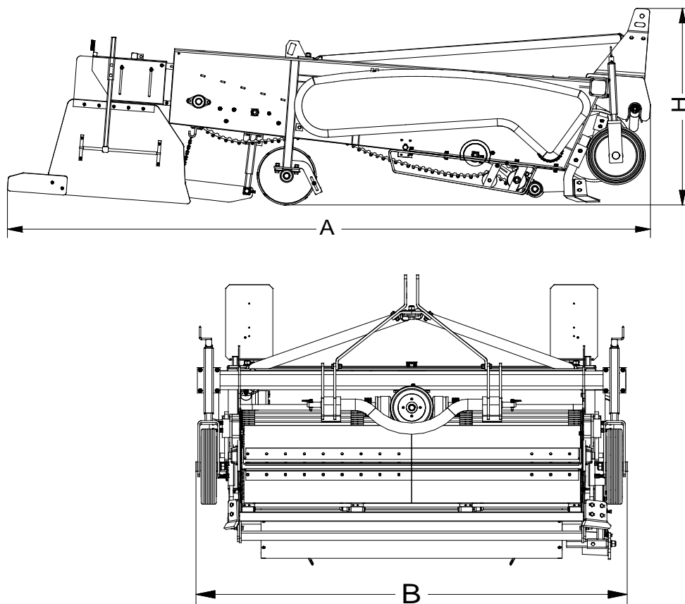
Rys. 5. Gabaryty w pozycji transportowej
