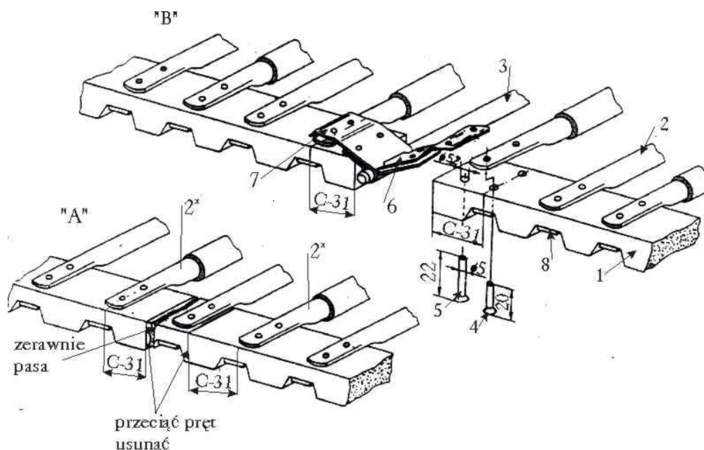
Rys. 10. Odsiewacz przenośnikowy
