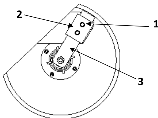
Rys. 6. Regulacja wysokości krojów.
