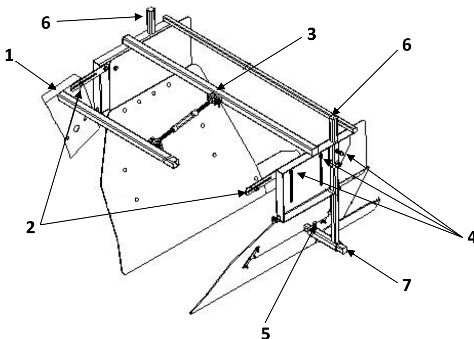
Rys. 8. Regulacja ustawienia formownicy
