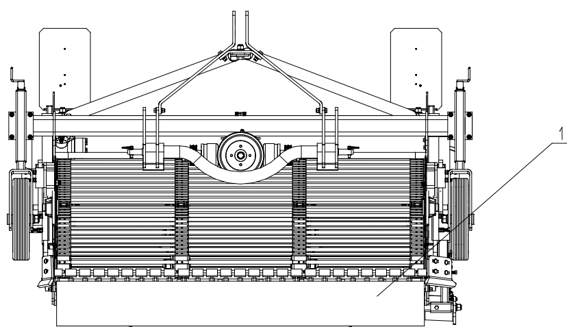
Rys.4b. Kopaczka PROFI z lemieszem listwowym.
