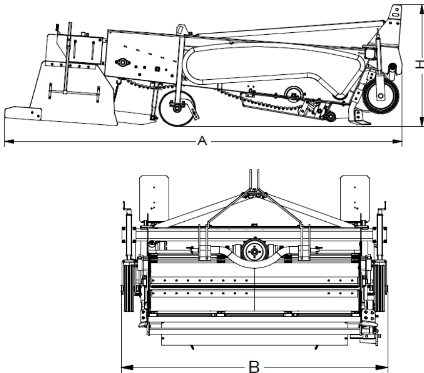
Gabaryty w pozycji transportowej
