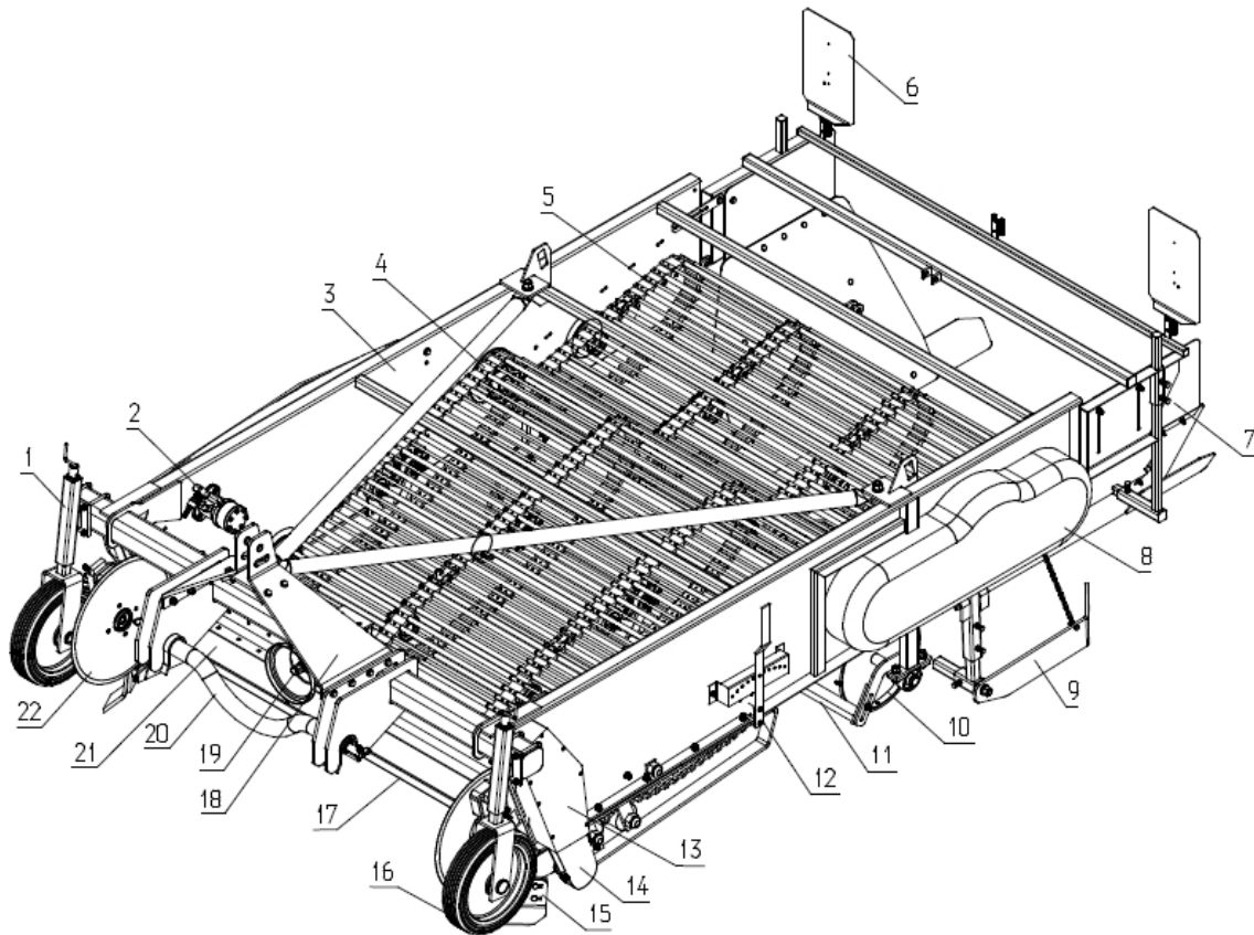
Rys.4a. Kopaczka PROFI z kwadratem kopiącym.
