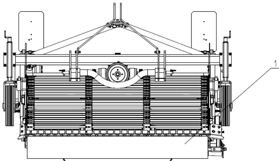
Rys.4b. Kopaczka PROFI z lemieszem listwowym.
