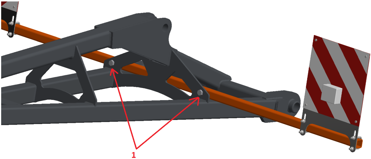
Rys. 4 Montaż oświetlenia na dyszu
