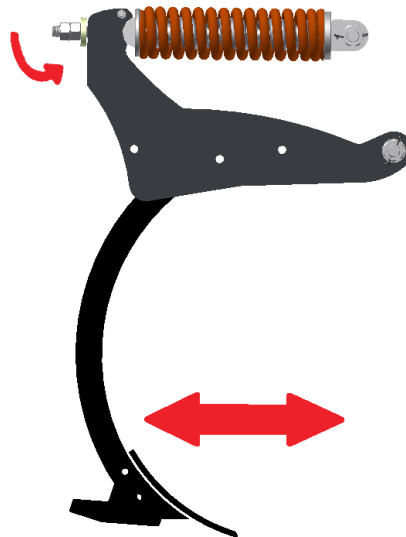
Rys. 14 Regulacja kąta natarcia grządzieli
