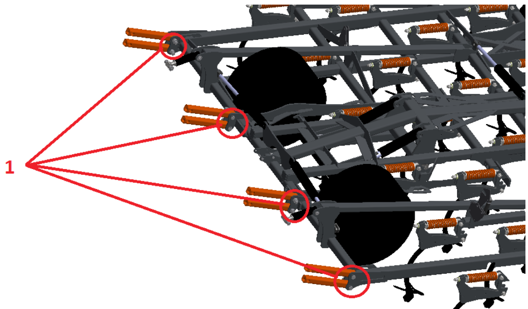
Rys. 5 Montaż ramion do ram
