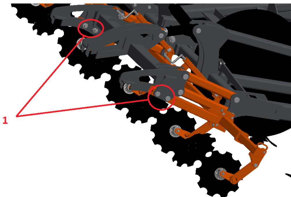
Rys. 7 Montaż belek z talerzami
