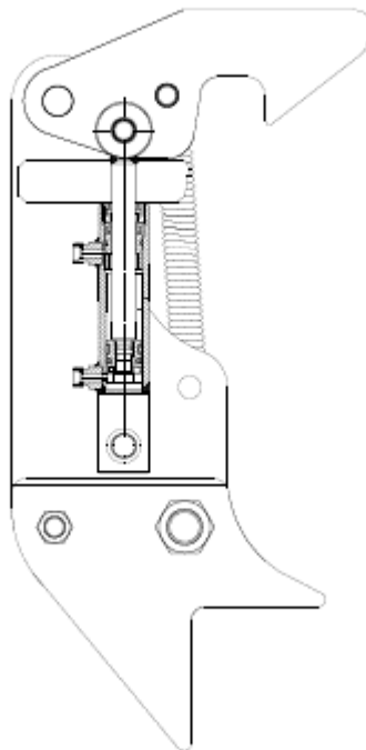
Rys. 12 Hydrauliczna blokada skrzydeł
