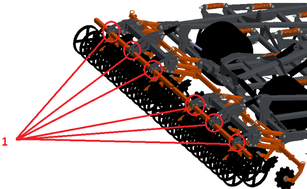
Miejsca mocowań zespołu wałów (nr 1)
