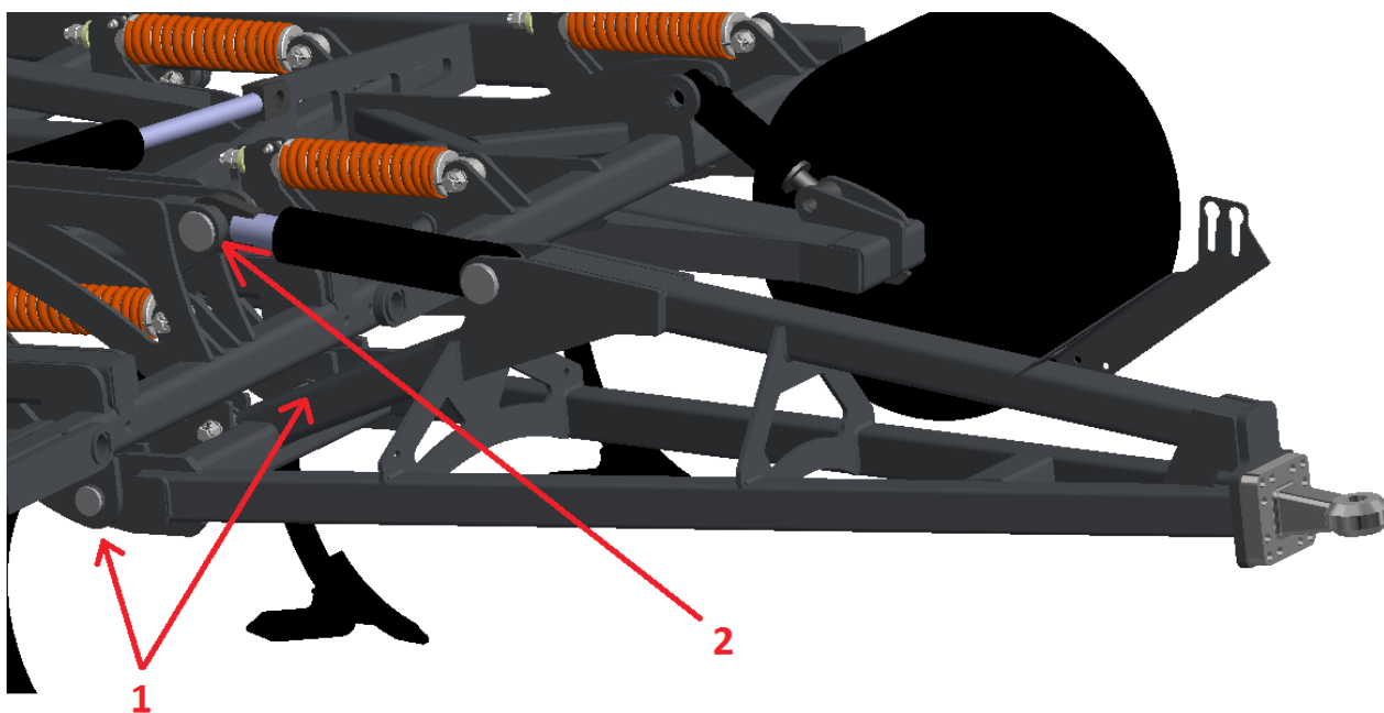
Rys.3 Montaż dyszla
