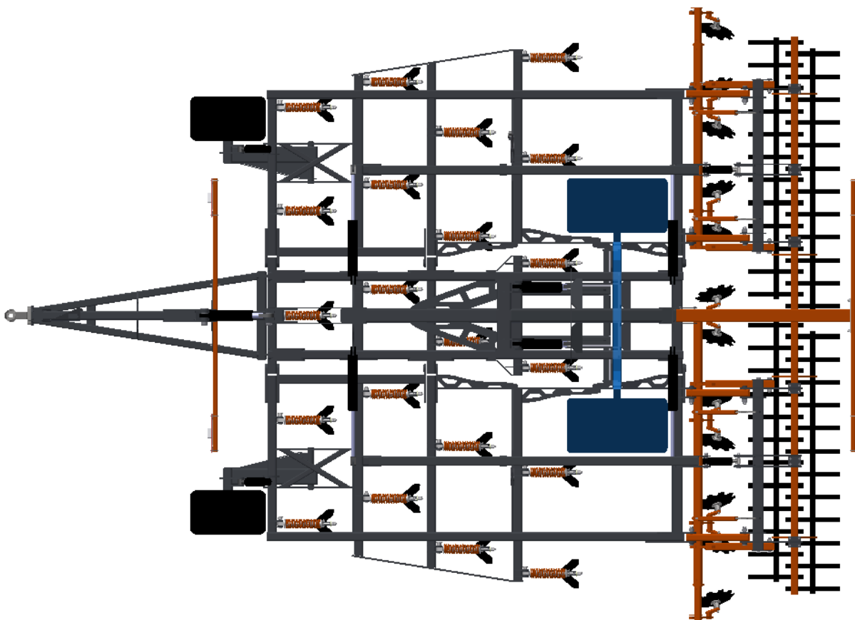
Rys. 17 Oś jezdna od góry
