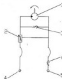
rys.26 Schemat podłączenia napędu hydraulicznego wentylatora
