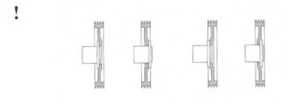
rys.18. Cztery sposoby montażu koła pasowego i kołnierza
