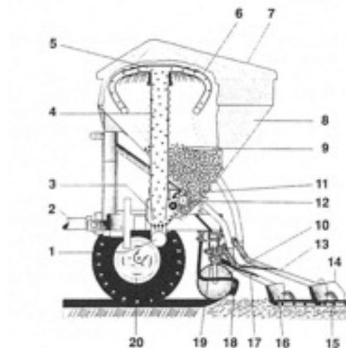
Rys.1 Schemat siewnika
