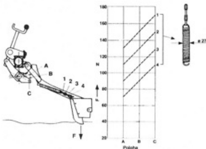
Rys.5 Wykres docisku na aparat wysiewczy
