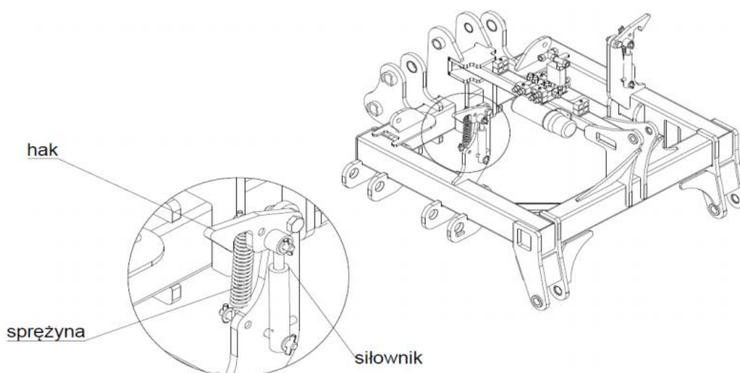
Rys. 4 Rama główna z mechanizmem automatycznej blokady skrzydeł.
