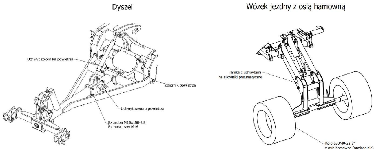
Rys. 14 Instalacja pneumatyczna osi hamownej
