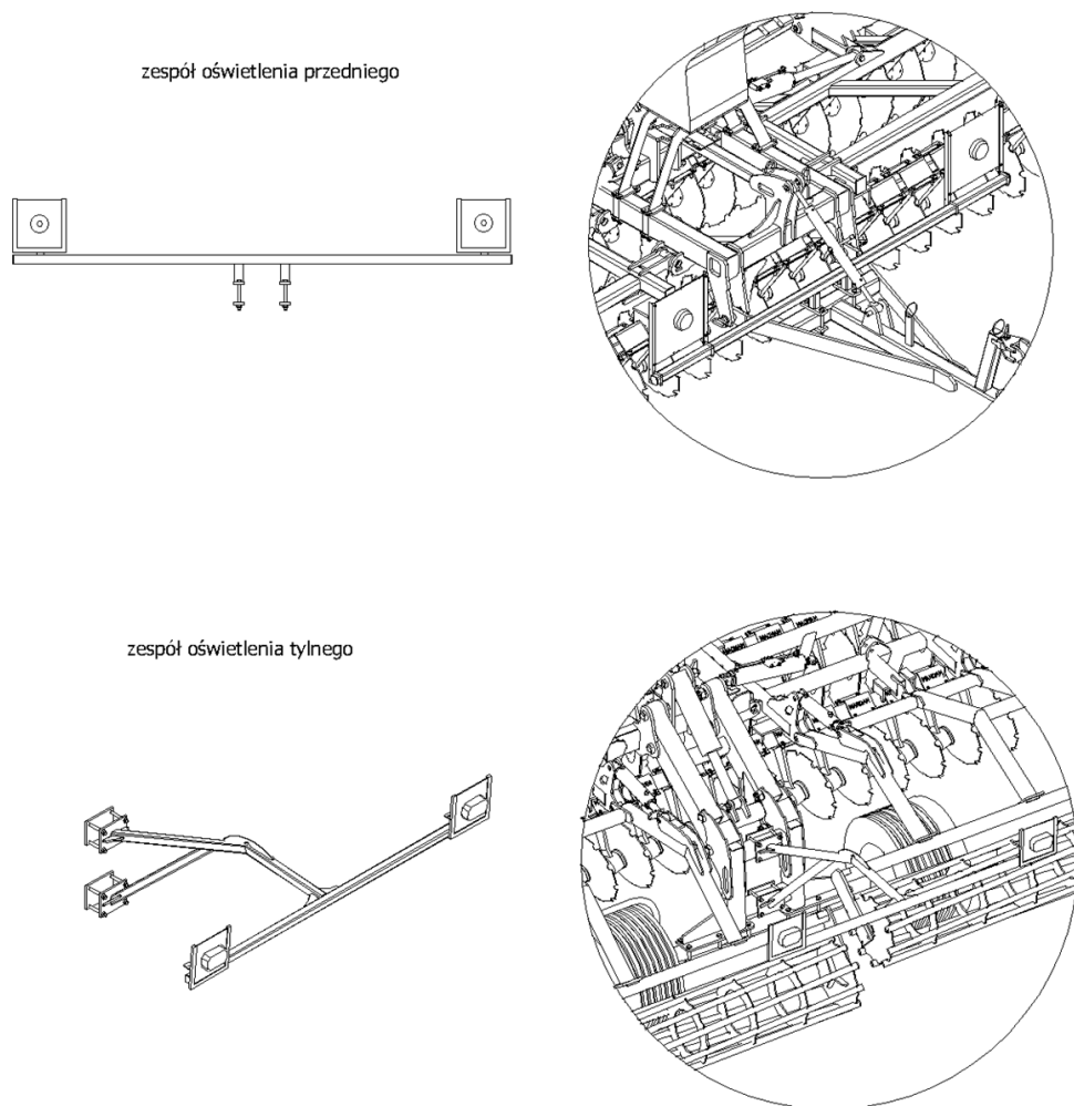
Rys. 13 Zespoły oświetlenia przedniego i tylnego oraz ich usytuowanie
