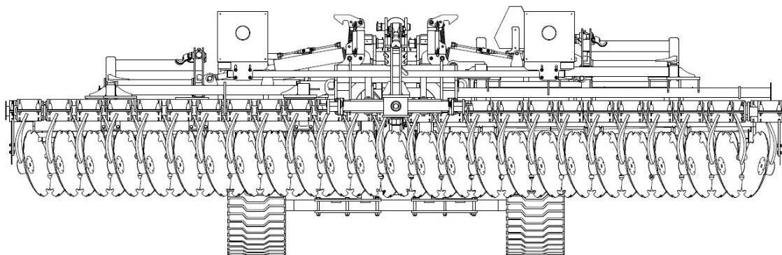
Rys. 8 Widok na maszynę w momencie zakończenia sekwencji otwierania skrzydeł. Ramiona maszyny są całkowicie otwarte.
