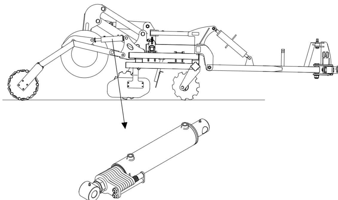
Rys. 10 Siłownik z zapadkami założonymi na tłoczysku w celu regulacji głębokości roboczej.
