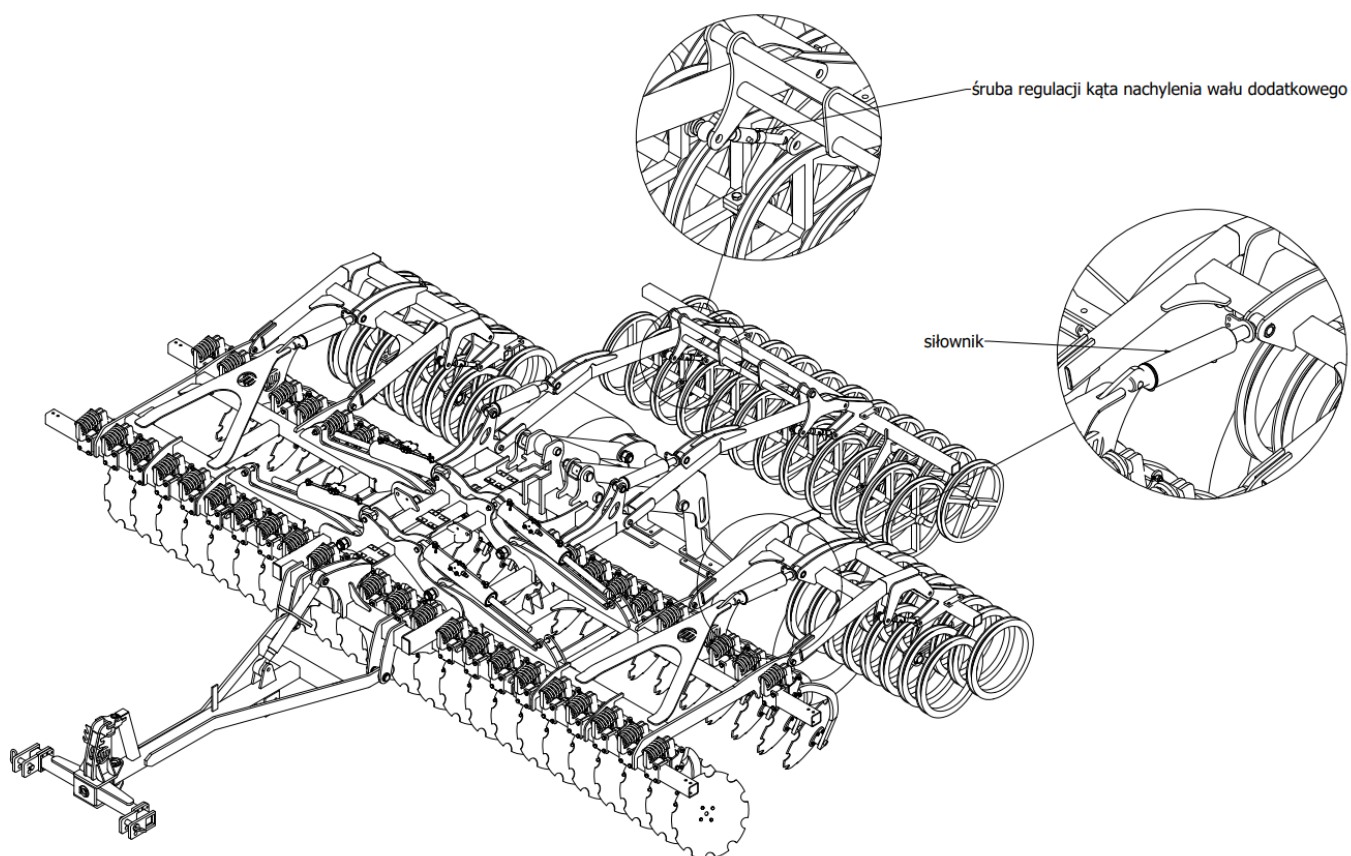
Rys. 9 Hydrauliczna regulacja głębokości wału.
