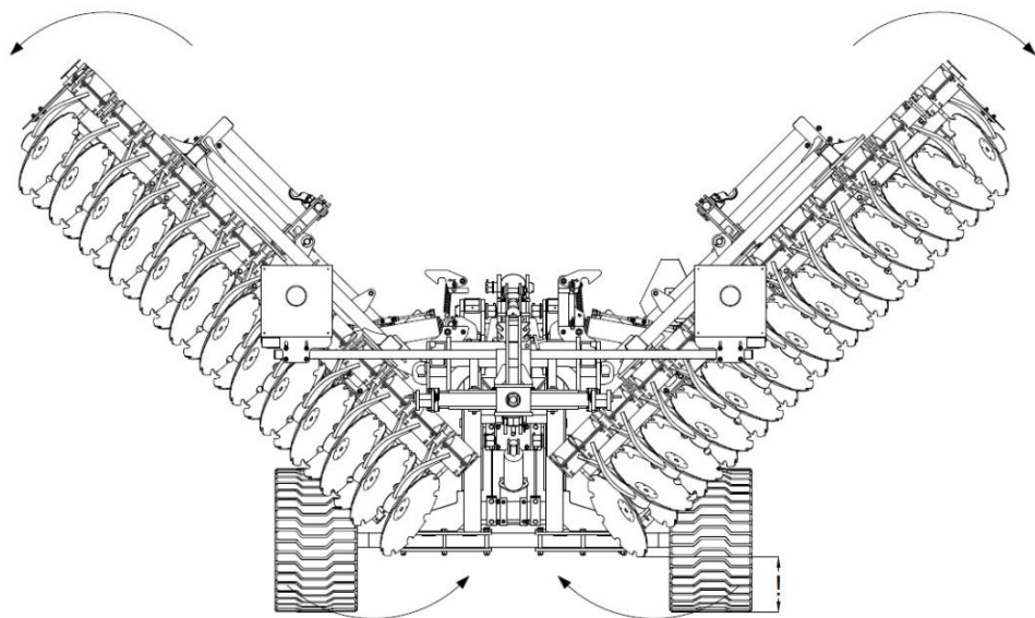
Rys. 7 Sekwencja otwierania maszyny: otwieranie maszyny ze zwróconą szczególną uwagą na wysokość końców ramion od podłoża.
