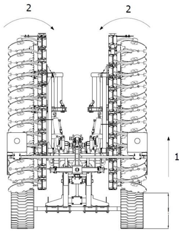
Rys. 5 Sekwencja otwierania maszyny: 1- podniesienie maksymalnie maszyny w górę, 2- złożenie skrzydeł maszyny do pozycji „zamkniętej”.
