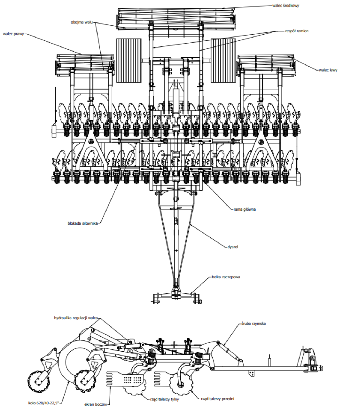
Rys.1 Brona talerzowa SAL-K
