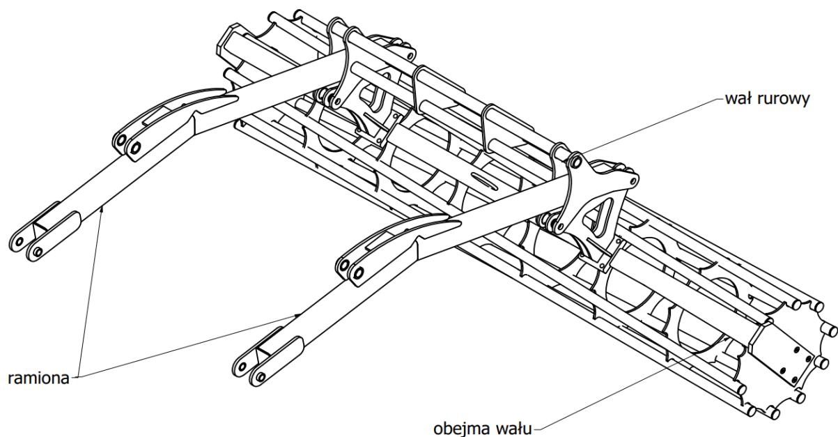
Rys. 2 Połączenie ramion z obejmą wału
