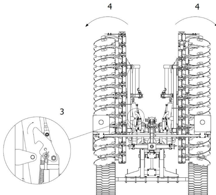
Rys. 6 Sekwencja otwierania maszyny: 3- uwolnienie haka mechanizmu hydraulicznej blokady skrzydeł 4- otwieranie skrzydeł maszyny.
