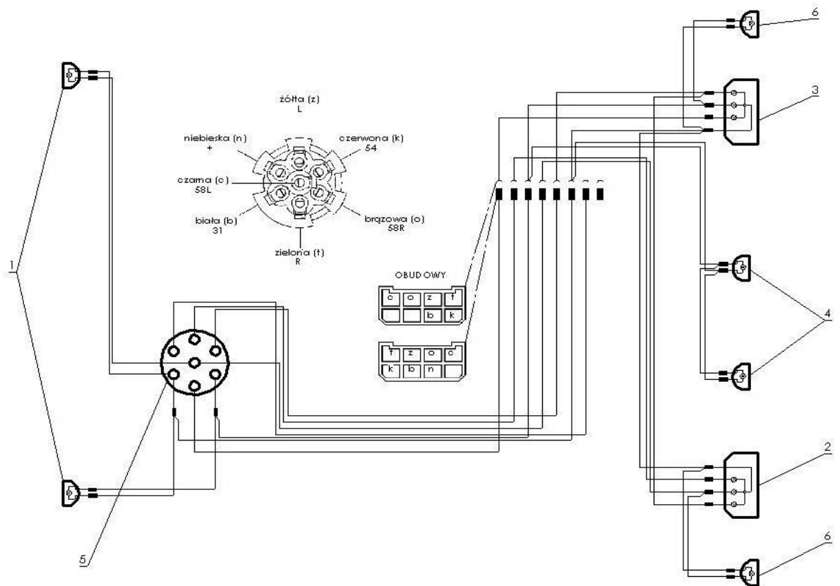
Rys. 10. Schemat instalacji elektrycznej przycepy.
