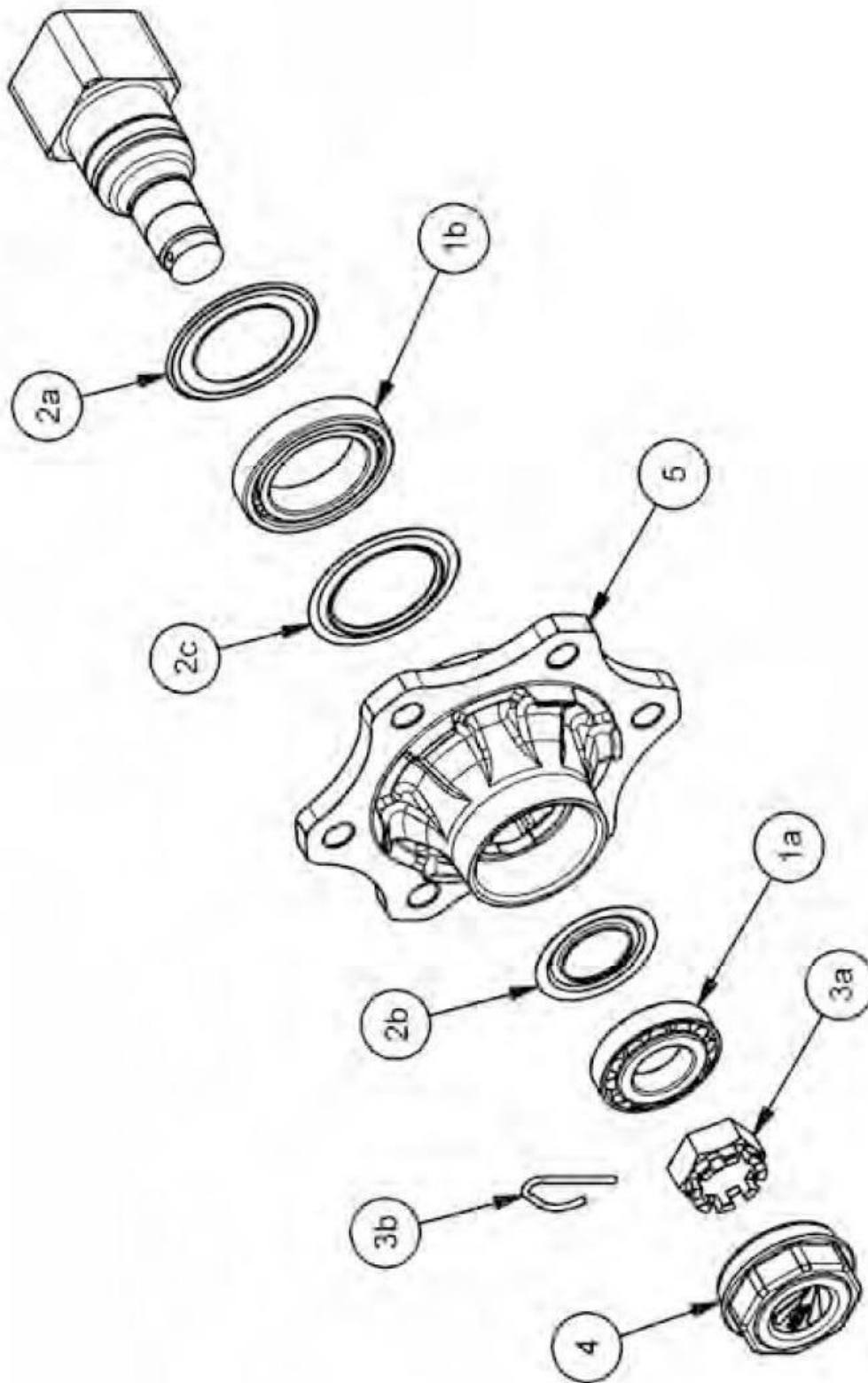
Rys. 24. Łożyskowanie osi jezdnej.
