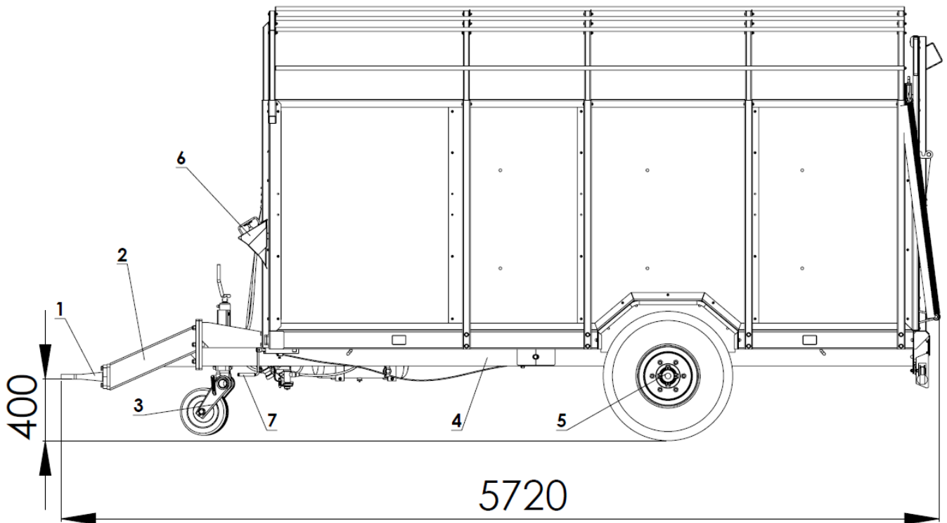
Rys. 2. Przyczepa T-677 (widok z boku).
