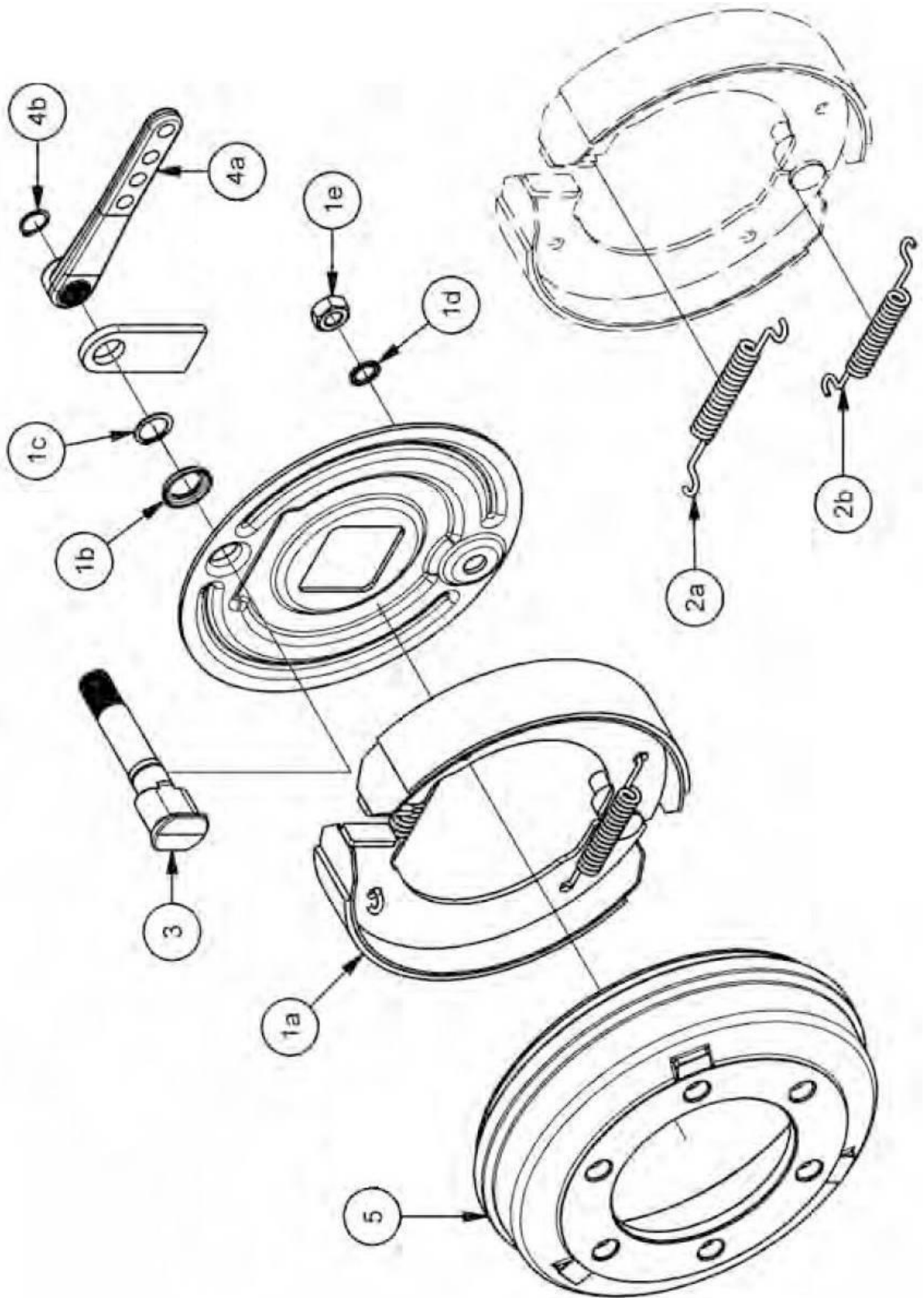
Rys. 25. Hamulec osi jezdnej.
