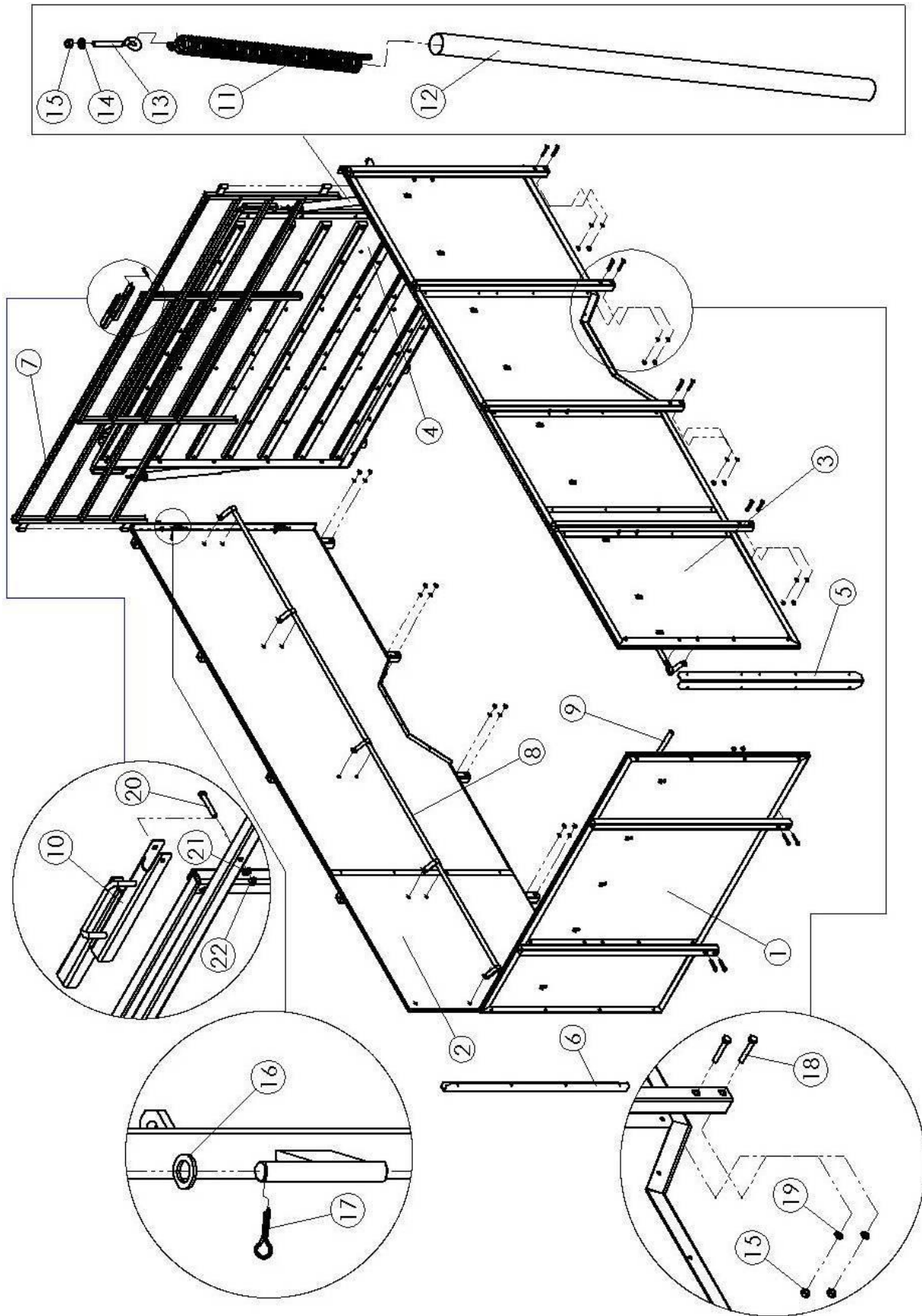
Rys. 16. Komplet ścian
