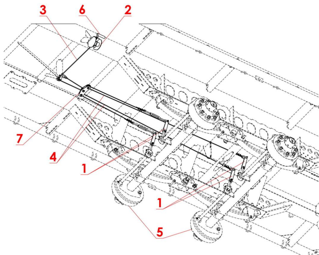
Rys. 8. Hamulec postojowy
