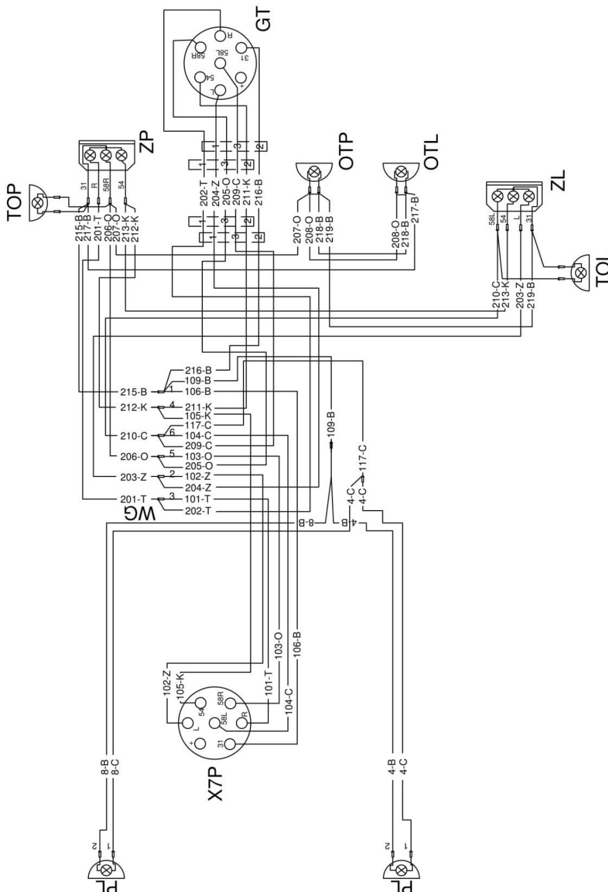
Rys. 9. Schemat instalacji elektrycznej przyczepty.
