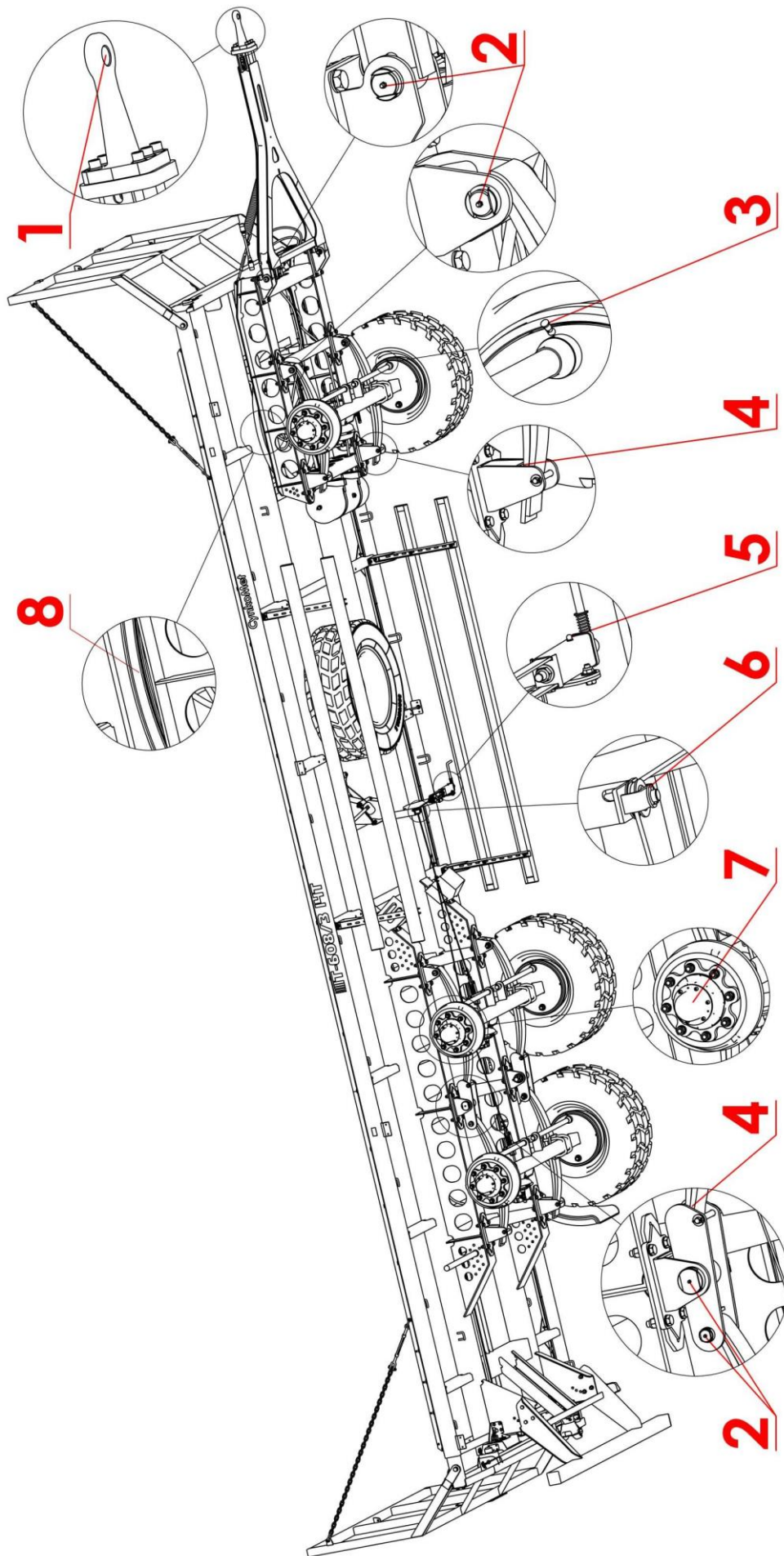
Rys. 13. Schemat smarowania
