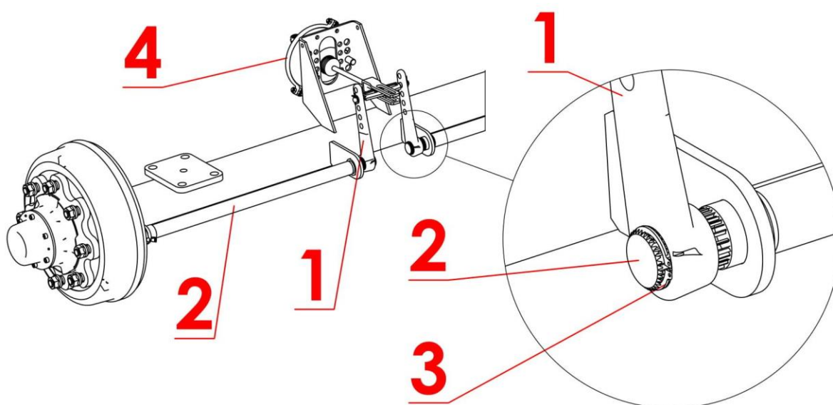
Rys. 11. Regulacja hamulców
