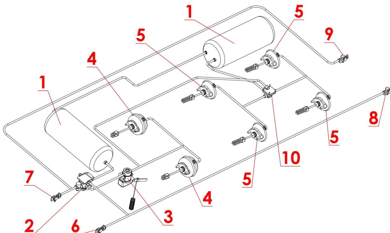
Rys. 6. Schemat pneumatycznej instalacji hamulcowej dwuprzewodowej.
