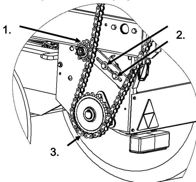
Rysunek 17. Napęd adaptera.
