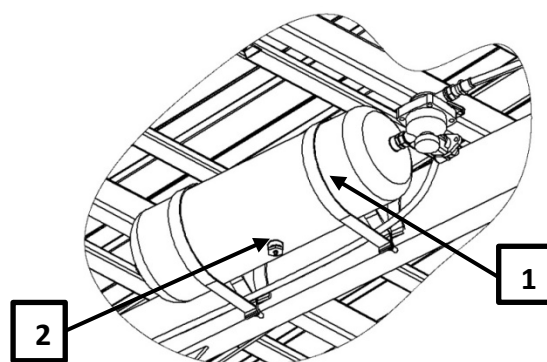
Rysunek 11. Odwadnianie zbiornika powietrza
