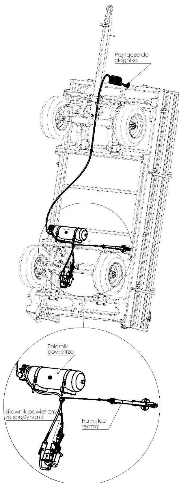
Rysunek 7. Schemat jednoobwodowej pneumatycznej instalacji układu hamulcowego.
