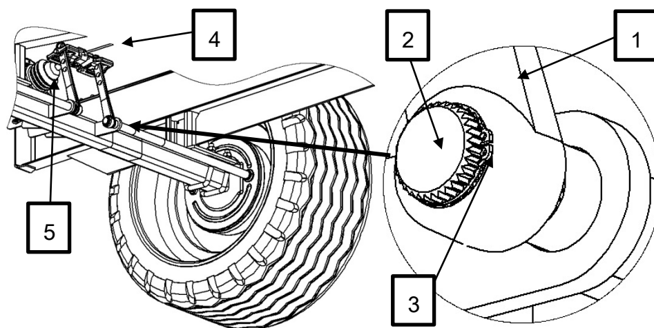
Rysunek 10. Regulacja hamulców
