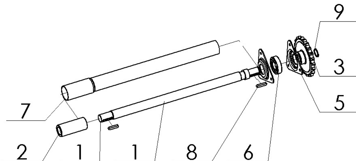
Tablica 7 Wałek 4 kpl.
