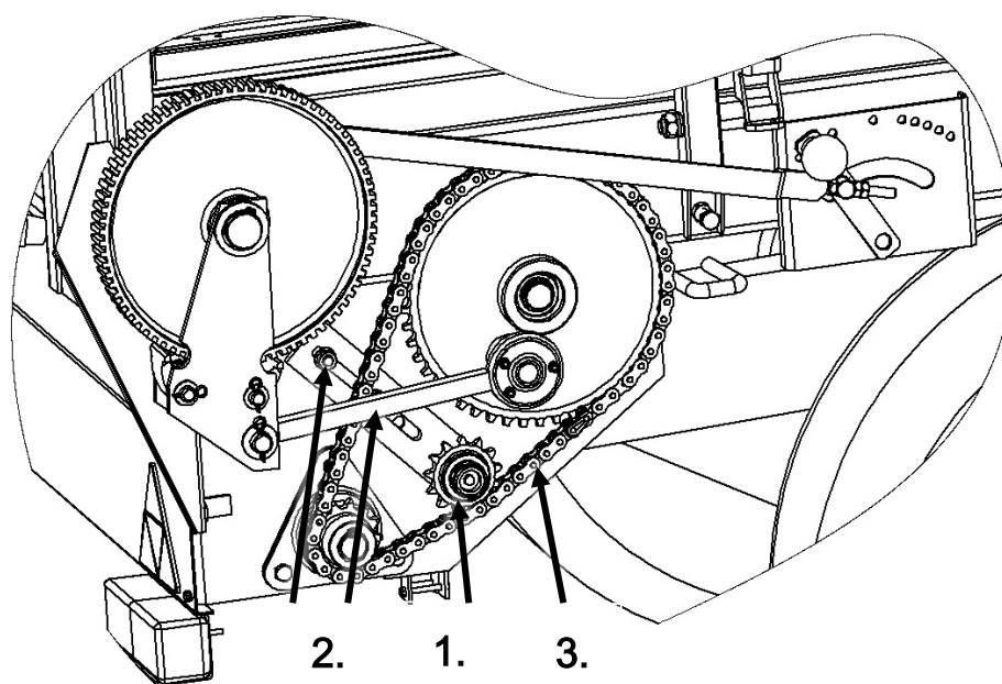
Rysunek 18. Napęd przenośnika podłogowego.
