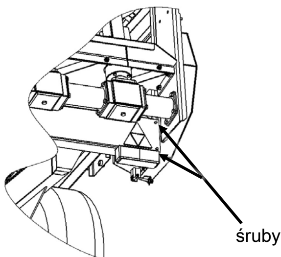
Rysunek 15. Umieszczenie śrub do odkręcenia osłony
