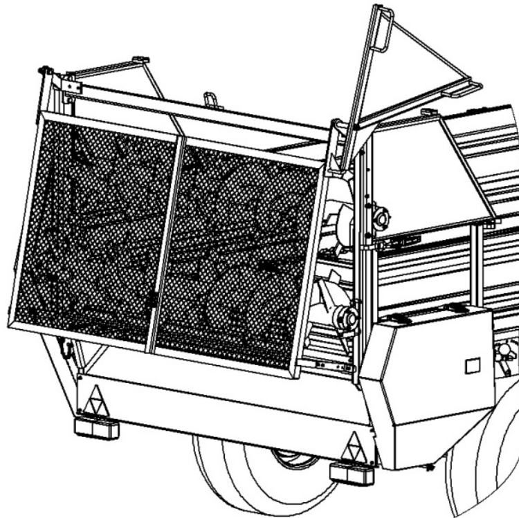
Rysunek 12. Zamontowana osłona.
