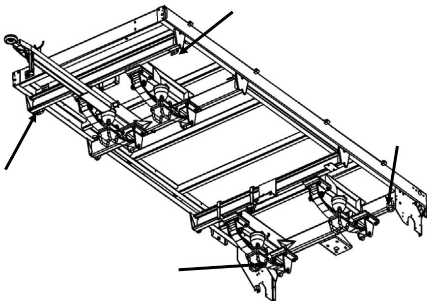
Rysunek 20. Uchwyty transportowe
