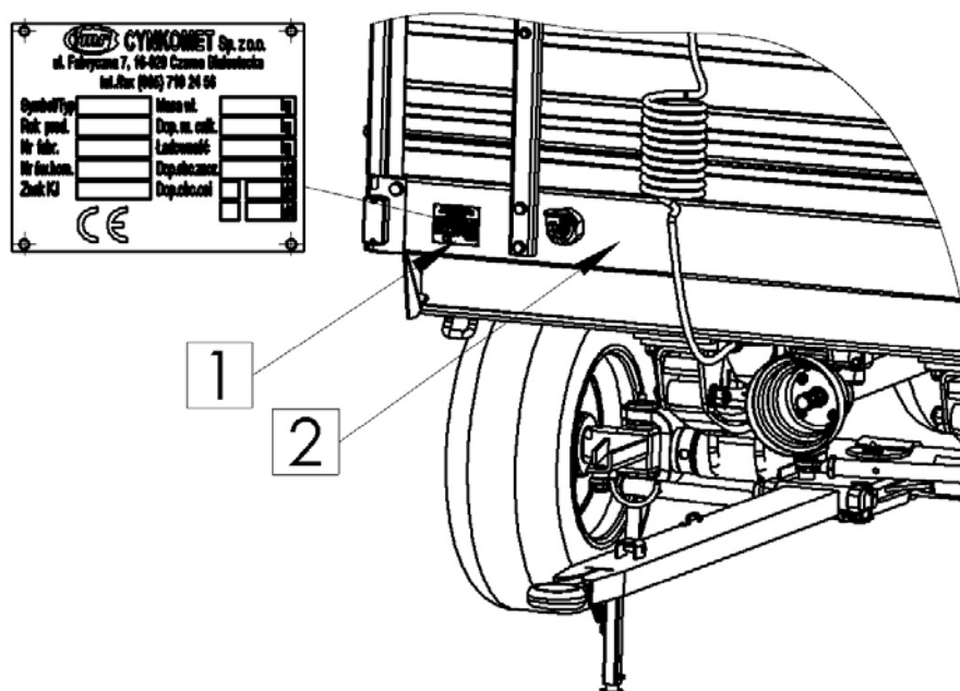
Rysunek 1. Miejsce umieszczenia tabliczki znamionowej i wybicia numeru fabrycznego
