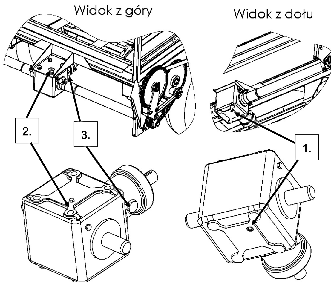
Rysunek 16. Skrzynia przekładniowa
