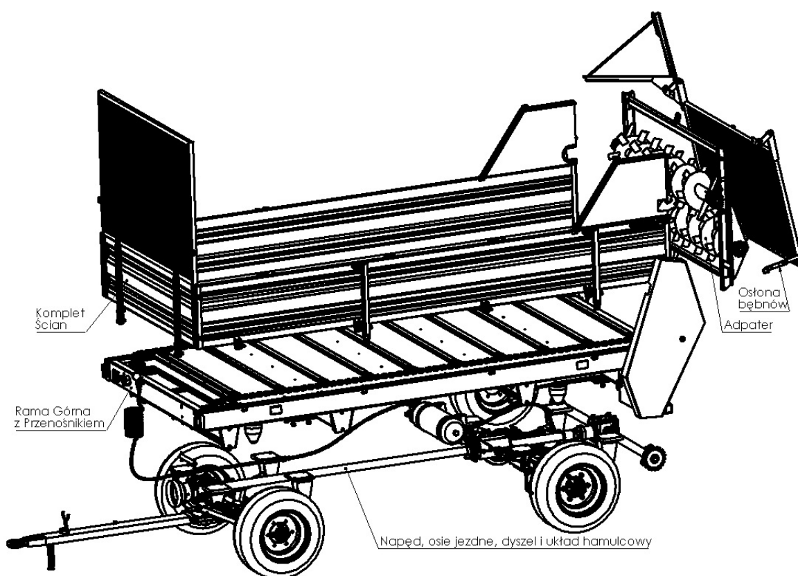
Rysunek 6. Budowa rozrzutnika.
