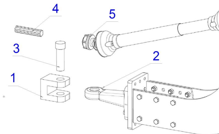
Rys. 24. Agregowanie ciągnika z opryskiwaczem
