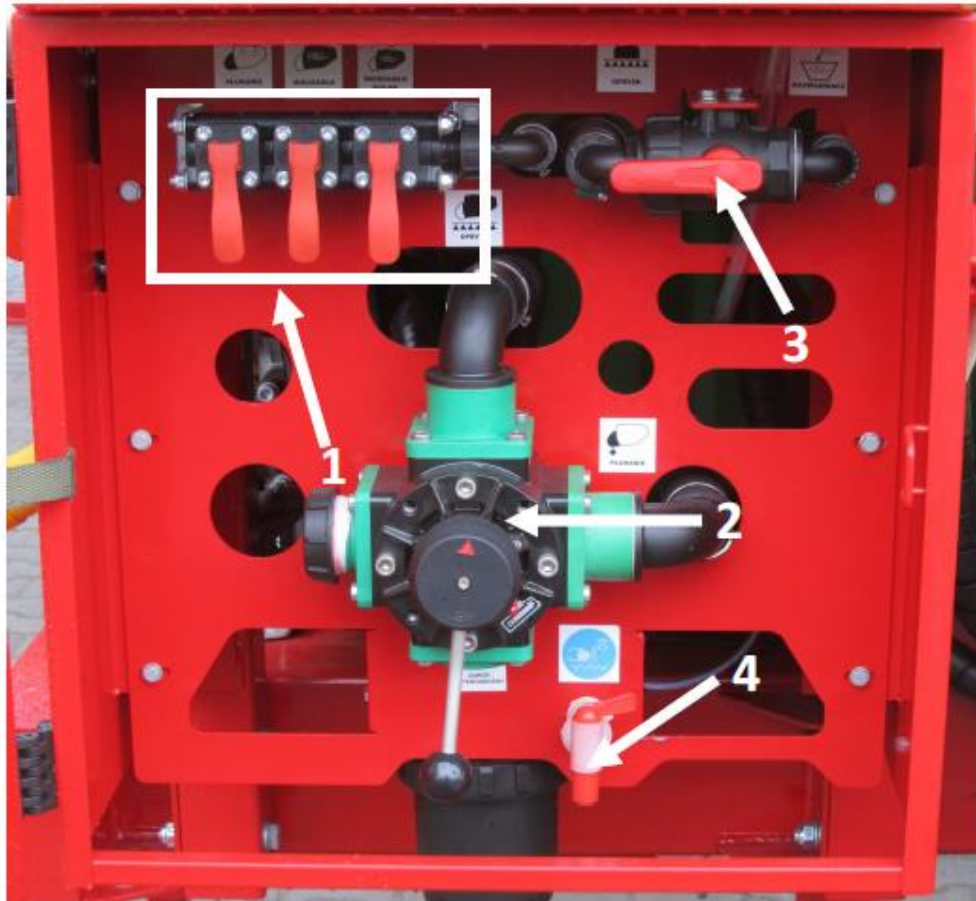
Rysunek 11 Pole obsługowe.
