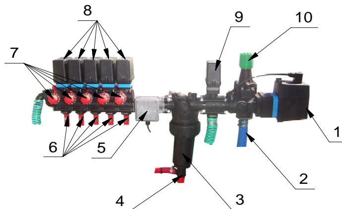
Rysunek 17 Zawór cieczowy sterowany elektrycznie
