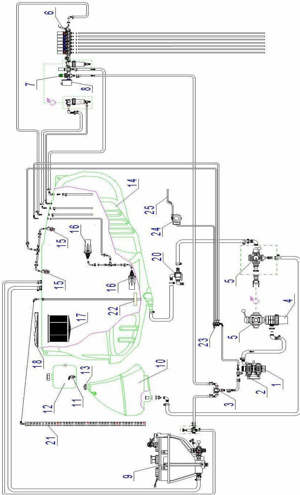
Rysunek 10 Schemat działania i obiegu cieczy opryskiwacza rolniczego GOLIAT 2500/3000 PHN.
