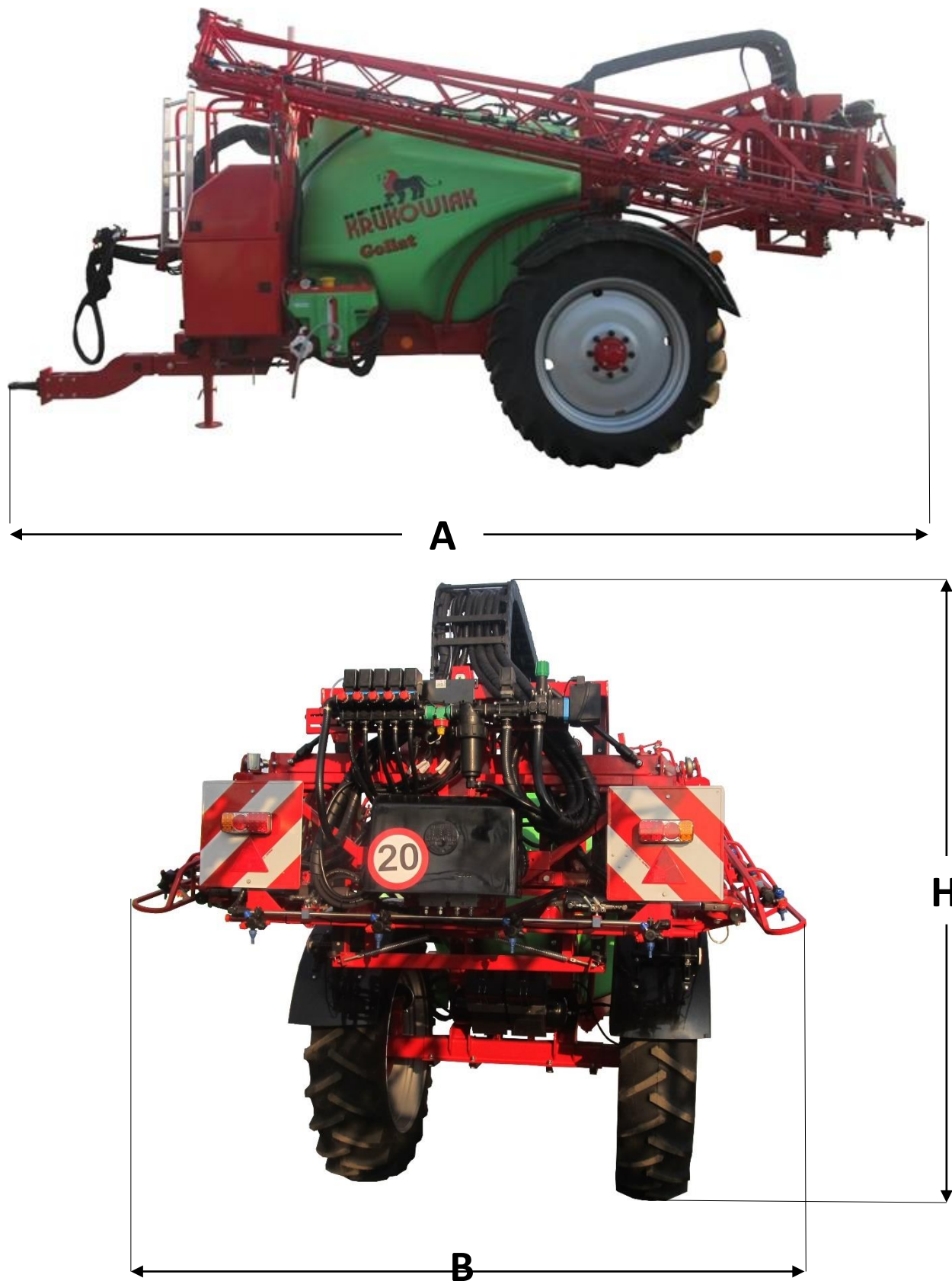
Rysunek 22 Gabaryty opryskiwacza GOLIAT 2500/3000 PHN w pozycji transportowej.
