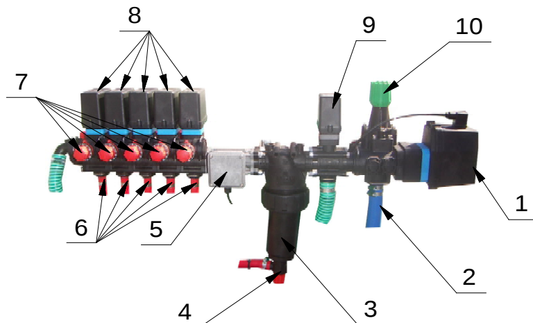
Rysunek 12 Zawór cieczowy sterowany elektrycznie
