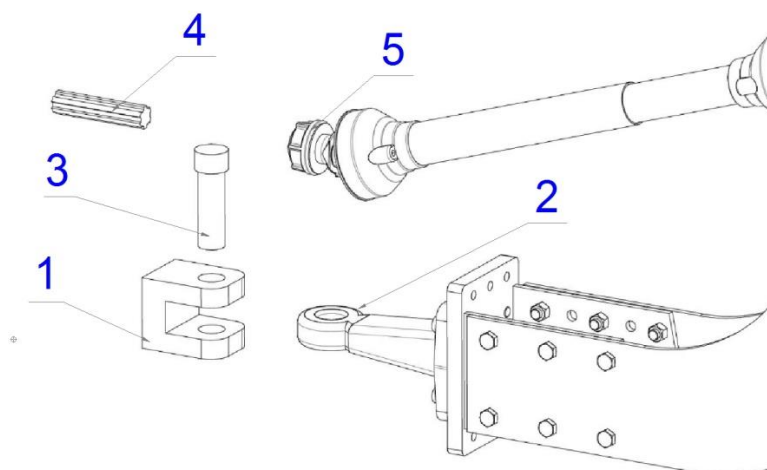
Rys. 20. Agregowanie ciągnika z opryskiwaczem
