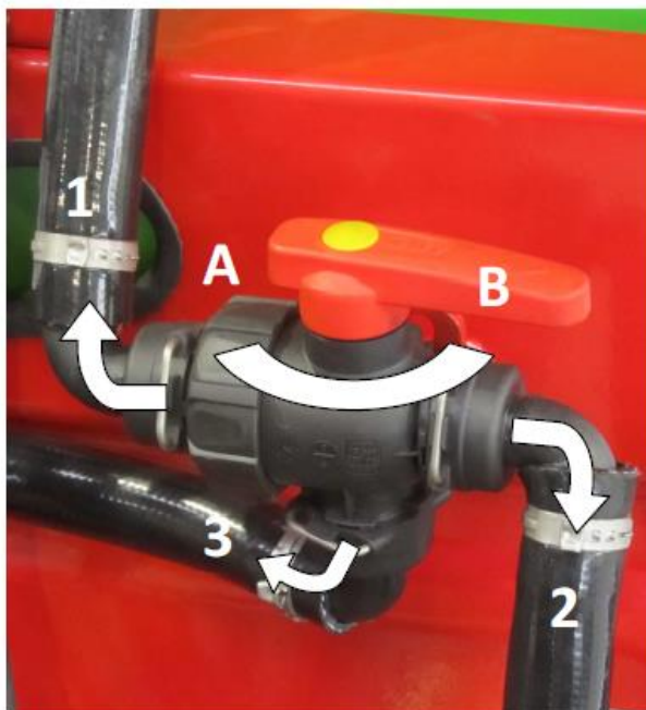
Rys. 10 Zawór kulowy.
