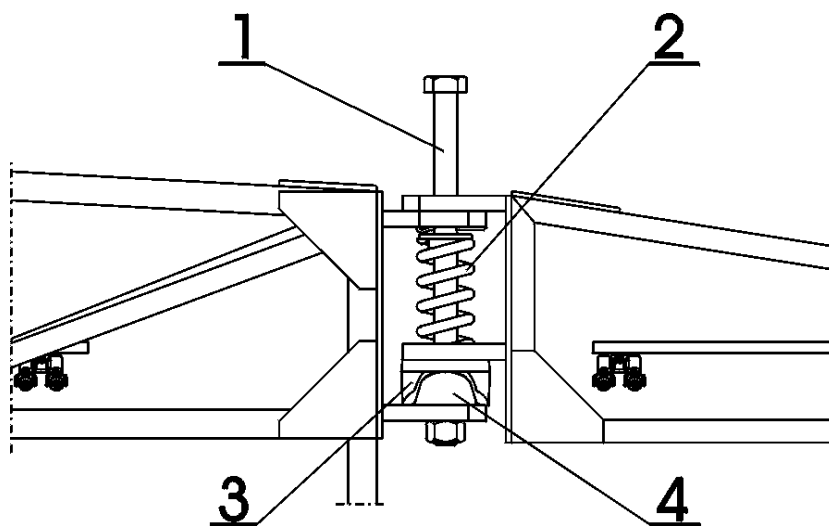
Rys. 6. Ogólny widok sprzęgła kłowego
