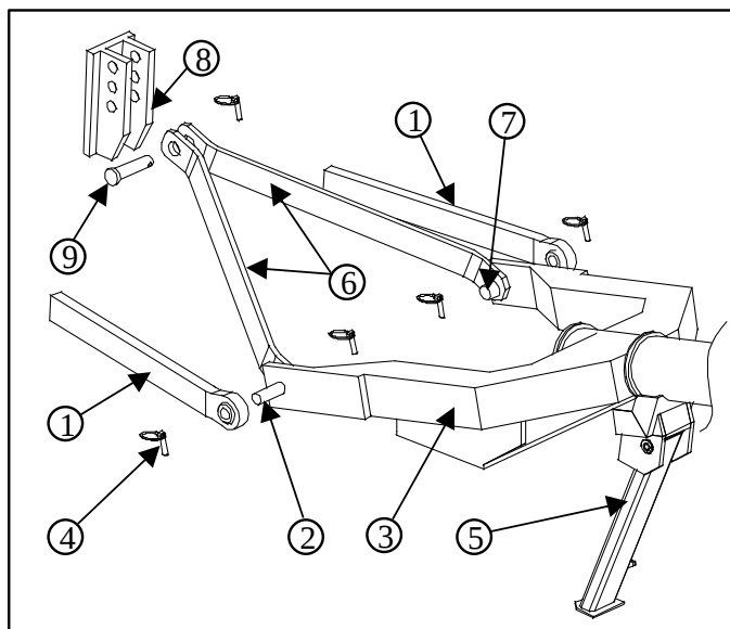
Rysunek 19 Agregowanie ciągnika z opryskiwaczem
