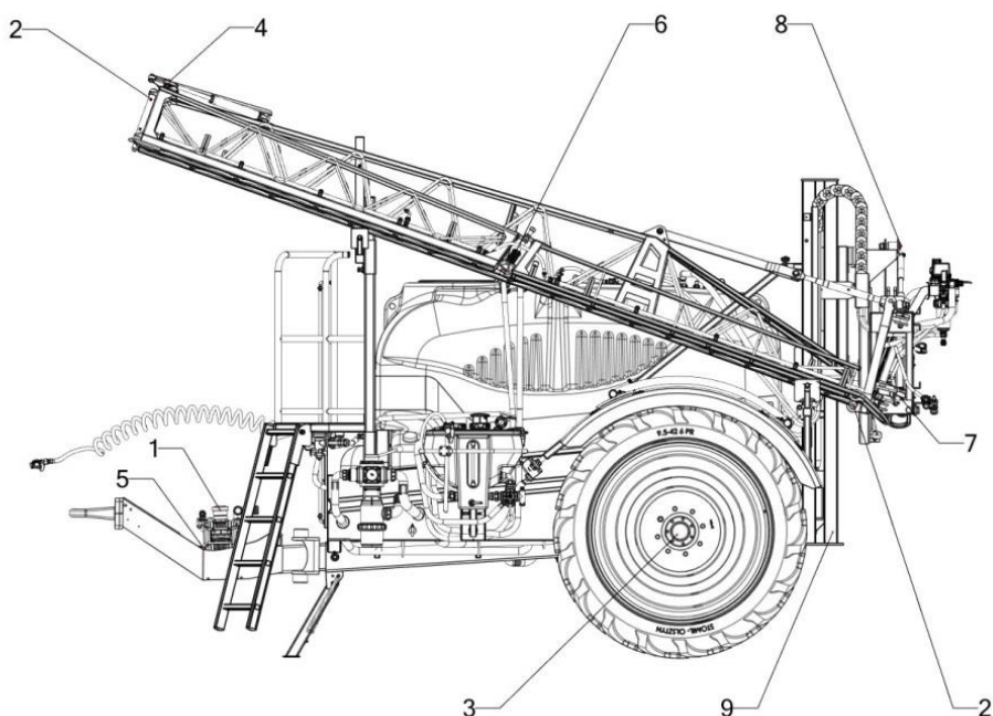
Rysunek 21. Punkty smarowania opryskiwaczy ORION 2500/3000 PHB.
