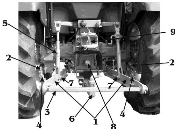
Rysunek 18 Ciągnik przygotowany do współpracy z opryskiwaczem
