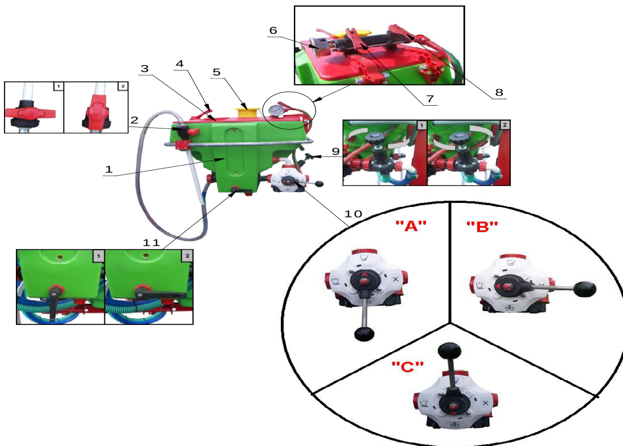
Rysunek 9 Budowa rozdzielacza bocznego POLMAC
