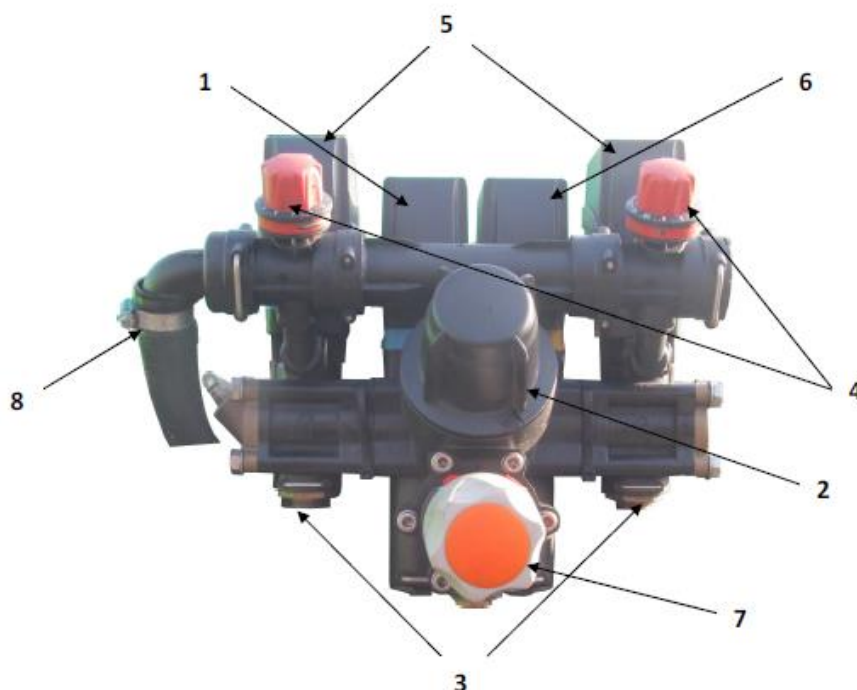
Rysunek 17 Zawór ciecowy sterowany elektrycznie
