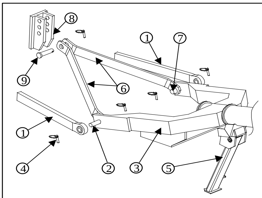
Rysunek 22 Agregowanie ciągnika z opryskiwaczem
