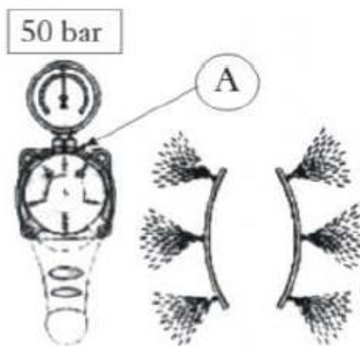
Rysunek 12 Przełączenie dźwigni przepływu cieczy w pozycję A.
