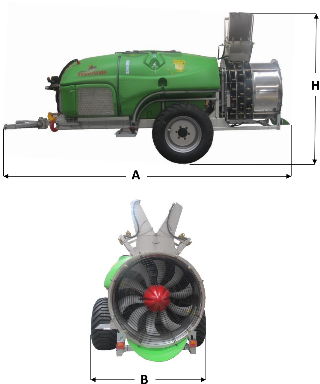
Rysunek 20 Gabaryty w pozycji transportowej
