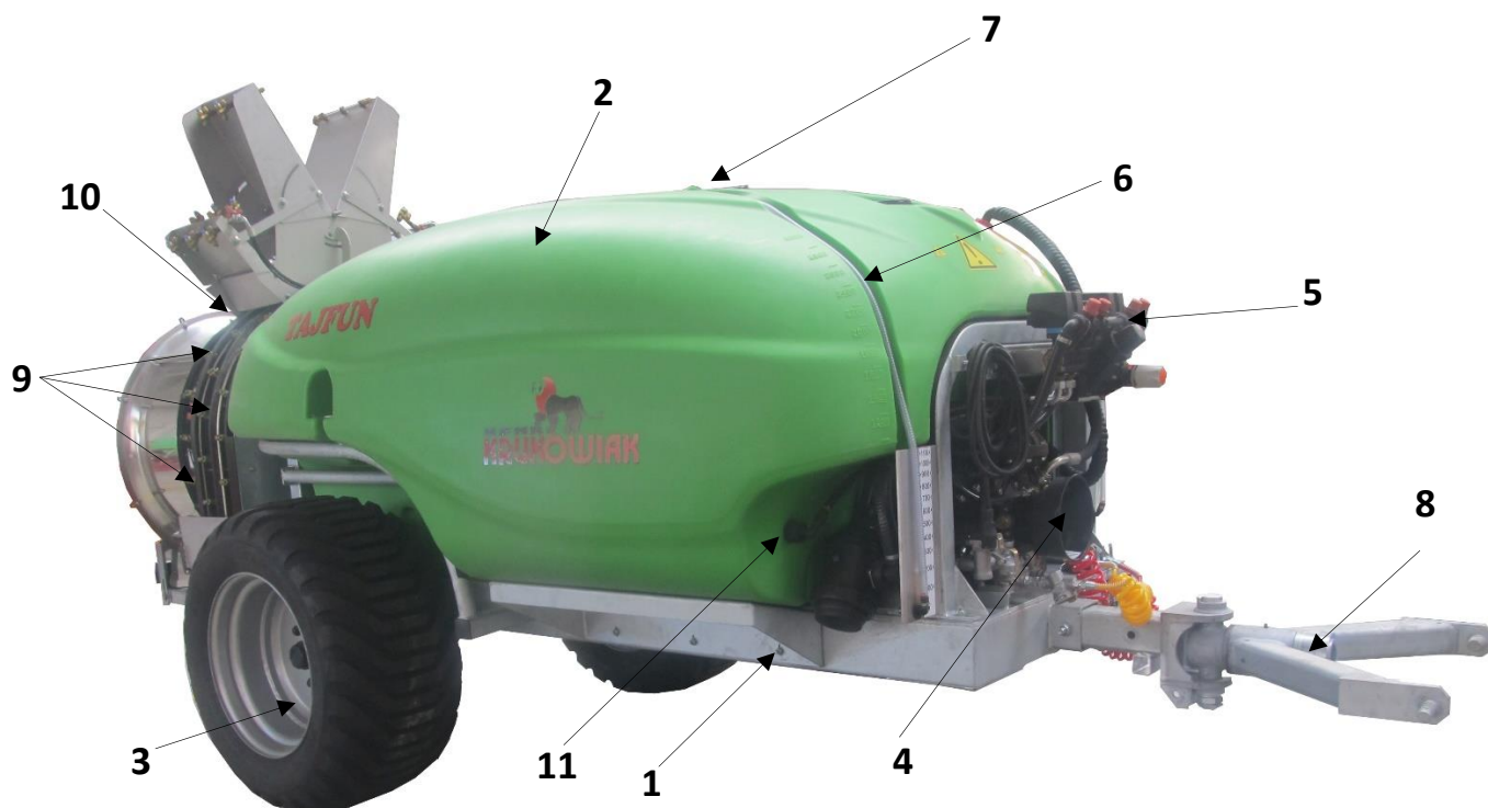
Rys. 4. Opryskiwacz sadowniczy przyczepiany TAIFUN.
