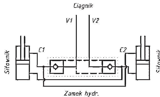
Rys. 6. Schemat instalacji hydraulicznej burty tylnej
