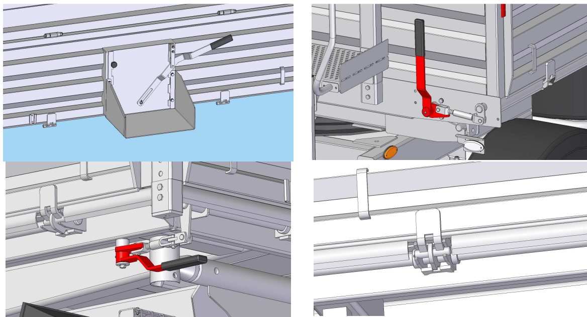
Rys. 7. Okno zsympowe i zamki burt skrzyni ładunkowej.
