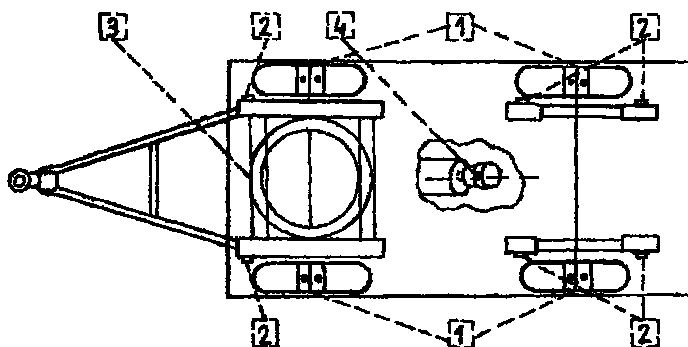
Rys.12. Punkty smarowania przyczep DB
