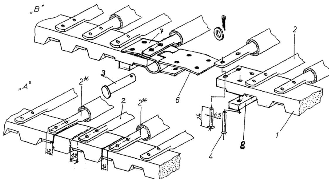
Rys. 23 - Odsiewacz przenośnikowy
