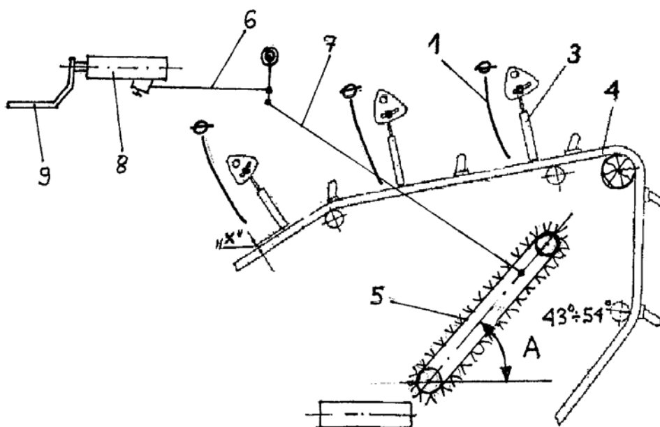
Rys. 15 - Oddzielacz łęcin
