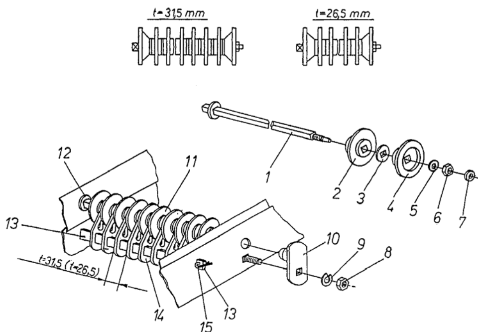
Rys. 21 - Odsiewacz tarczowy
