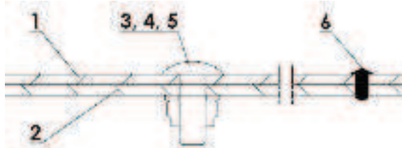
Rysunek 4.2. Sposób łączenia podłogi i ramy górnej (wersja cynkowana ogniowo).
