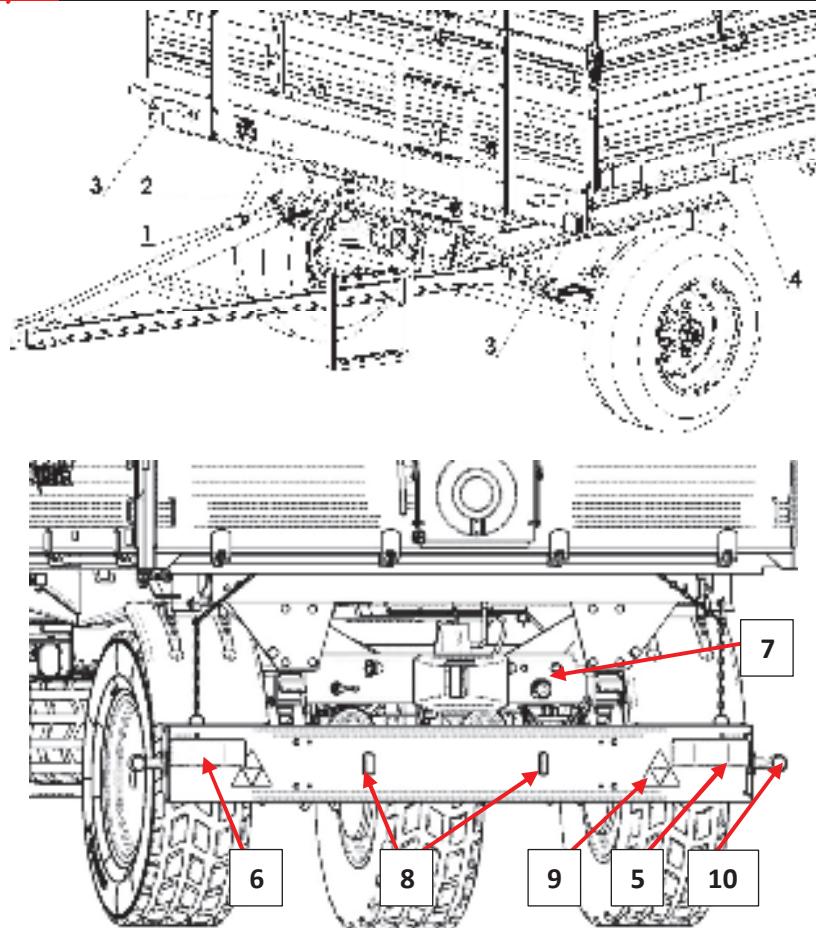
Rys. 13. Schemat układu oświetlenia i sygnalizacji
