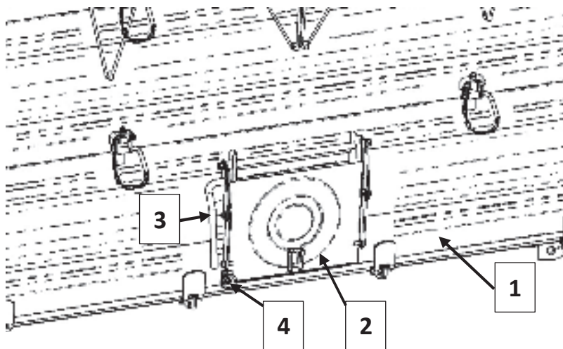
Rysunek 7. Okno zsypowe.
