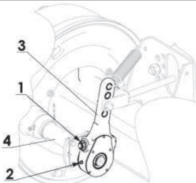
Rysunek 6.5. Regulacja hamulców
