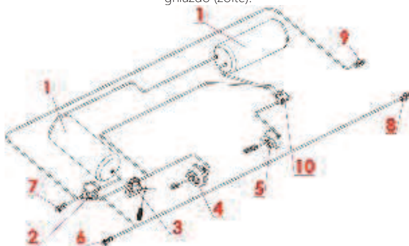
Rysunek 9.2. Schemat pneumatycznej instalacji hamulcowej dwuprzewodowej z automatycznym regulatorem siły hamowania
