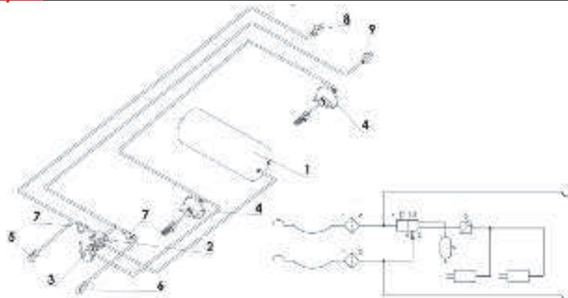
Rysunek 9.1. Schemat pneumatycznej instalacji hamulcowej dwuprzewodowej.
