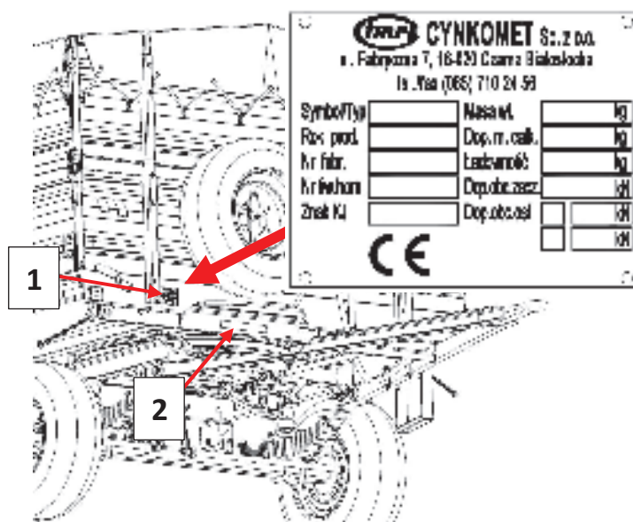
Rysunek 1. Miejsce umieszczenia tabliczki znamionowej i wybicia numeru fabrycznego (homologacja PL).
