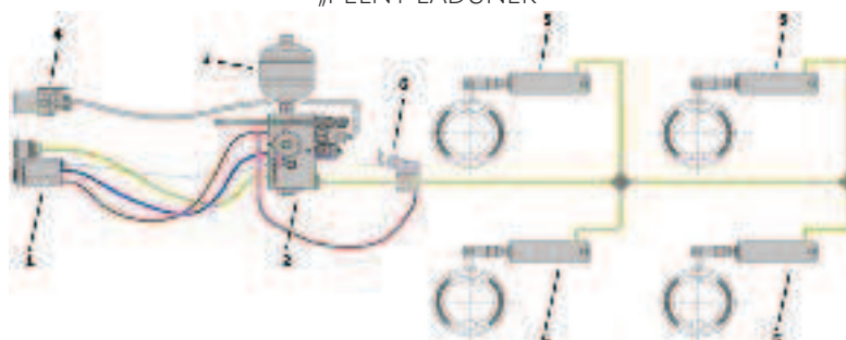
Rysunek 4.8. Schemat hydraulicznej instalacji hamulcowej.
