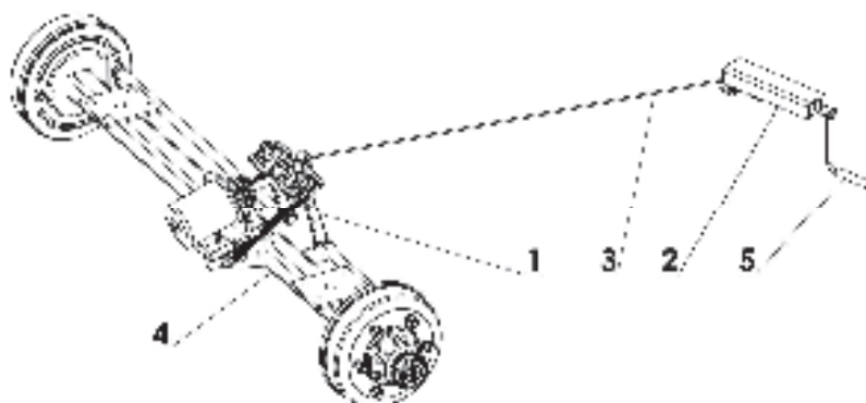
Rys. 11. Hamulec postojowy
