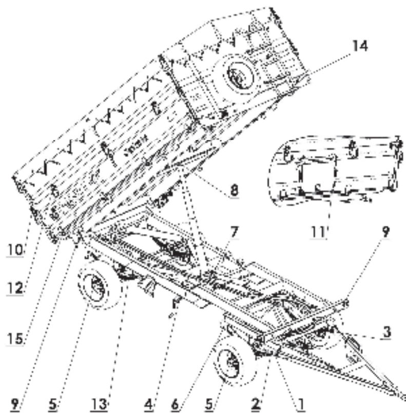
Rys. 20. Schemat smarowania
