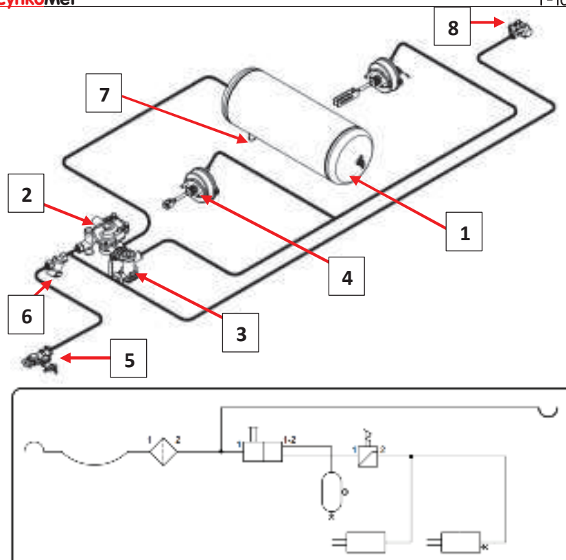
Rys. 9. Schemat pneumatycznej instalacji hamulcowej jedнопrzewodowej.
