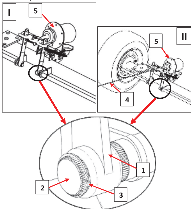
Rys. 17. Regulacja hamulców
