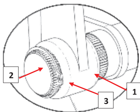
Rys. 18. Regulacja hamulców
