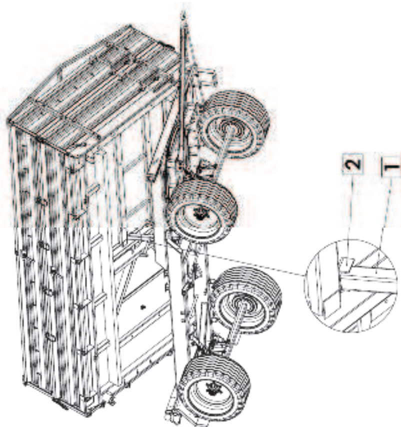
Rys. 17. Sposób podparcia skrzyni ładunkowej
