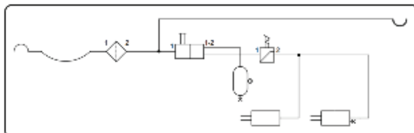
Rys. 9. Schemat pneumatycznej instalacji hamulcowej jedнопроводowej.
