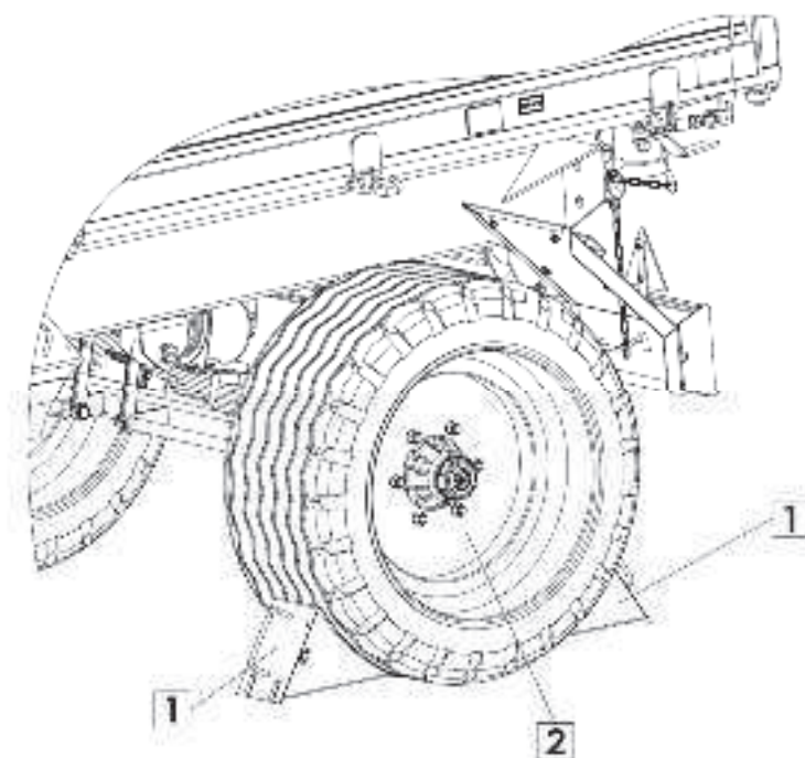
Rysunek 3. Sposób ustawiania klinów.
