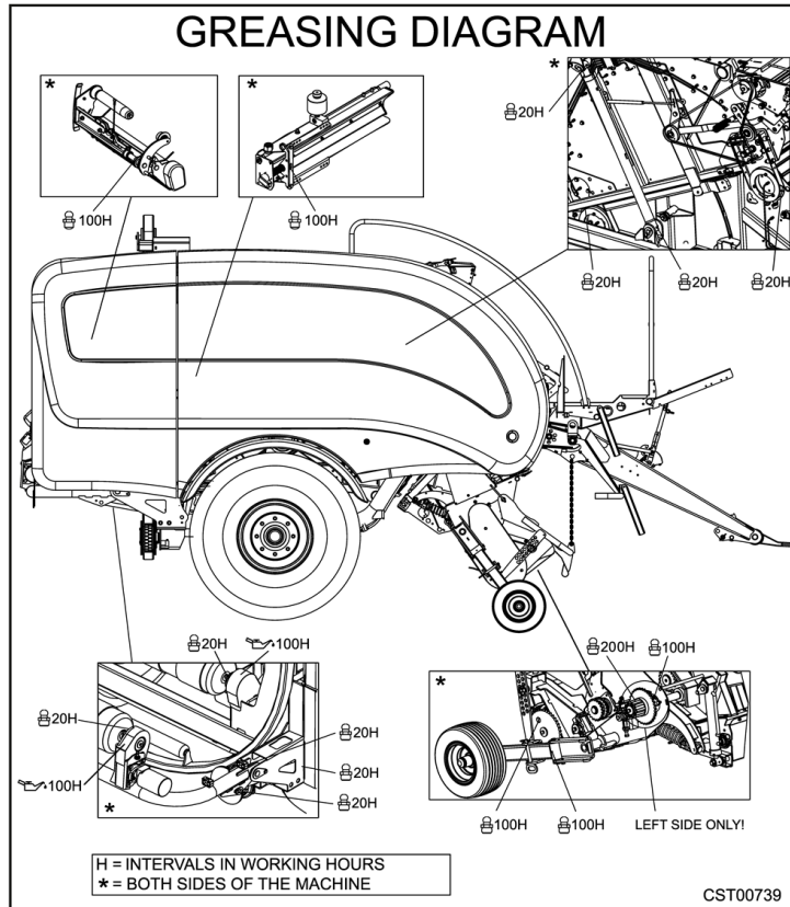
Schemat smarowania
