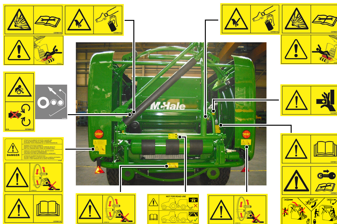
Etykiety z tyłu urządzenia
