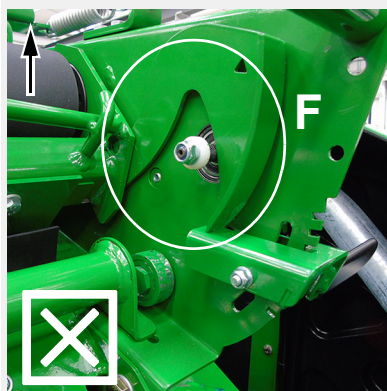
Nóż niezakleszczony (reset)
