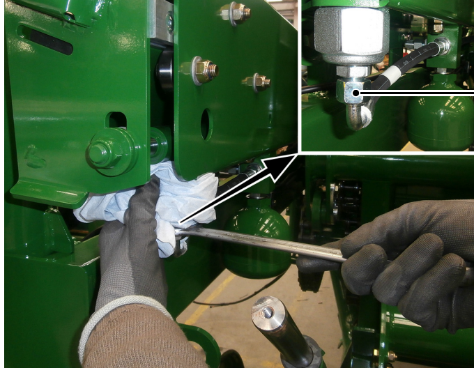
Przewód ciśnieniowy akumulatora
