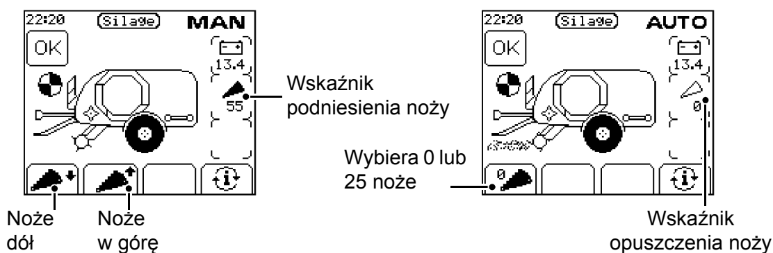
Obsługa noży standardowych
