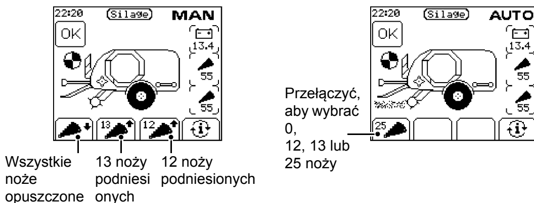
Obsługa wyboru noży
