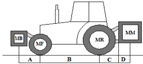
Rys.33. Określenie stateczności statecznej
