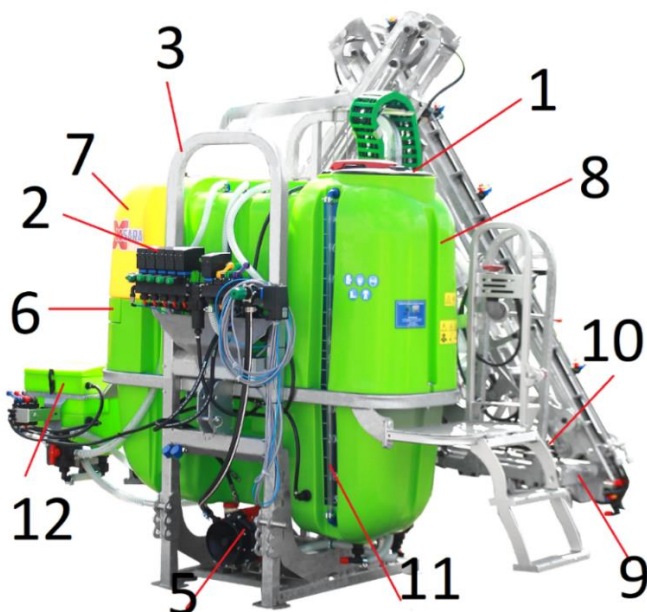
Rys.2. Budowa opryskiwacza zawieszanego typu Xsara.
