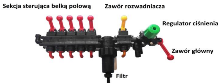
Rys.22.Budowa rozdzielacza.
